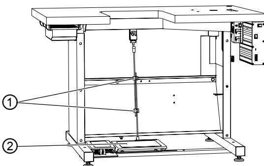
Afb. 57: Pedaal instellen
