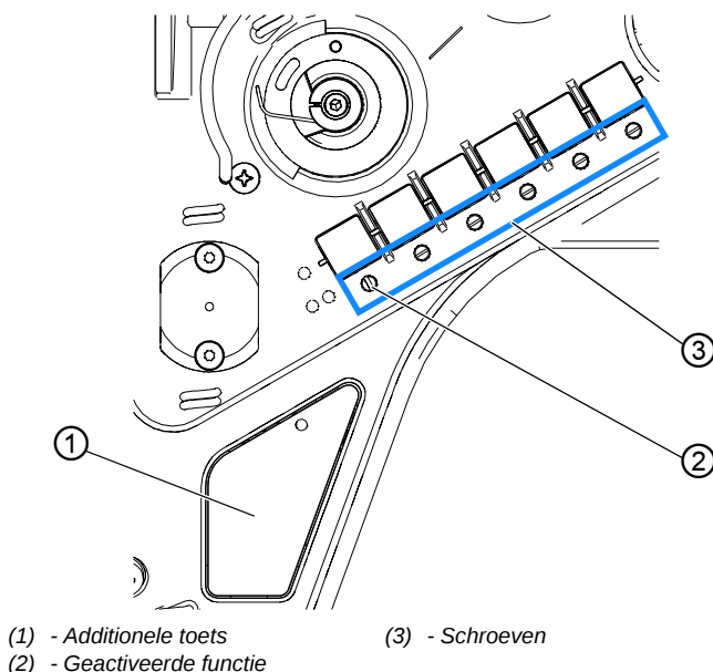
Afb. 35: Toetsfunctie overbrengen naar de additionele toets.
