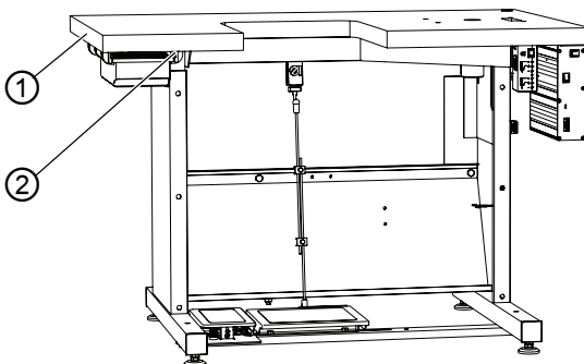
Afb. 56: Werkhoogte instellen
