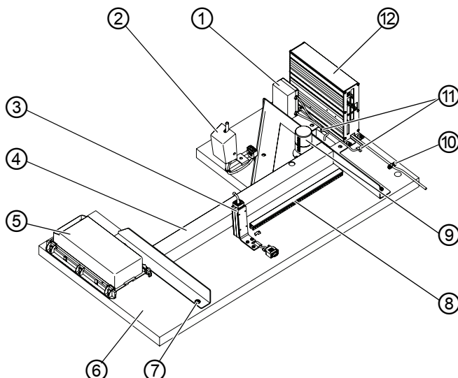
Afb. 50: Machines met een standaardarm
