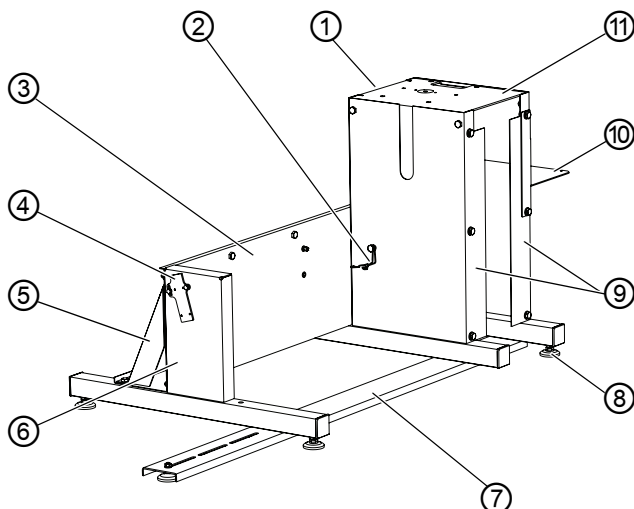
Afb. 48: Onderstel voor machines met een lange arm
