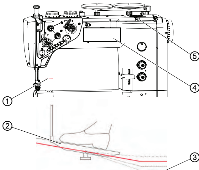
Afb. 36: Draad afsnijden
