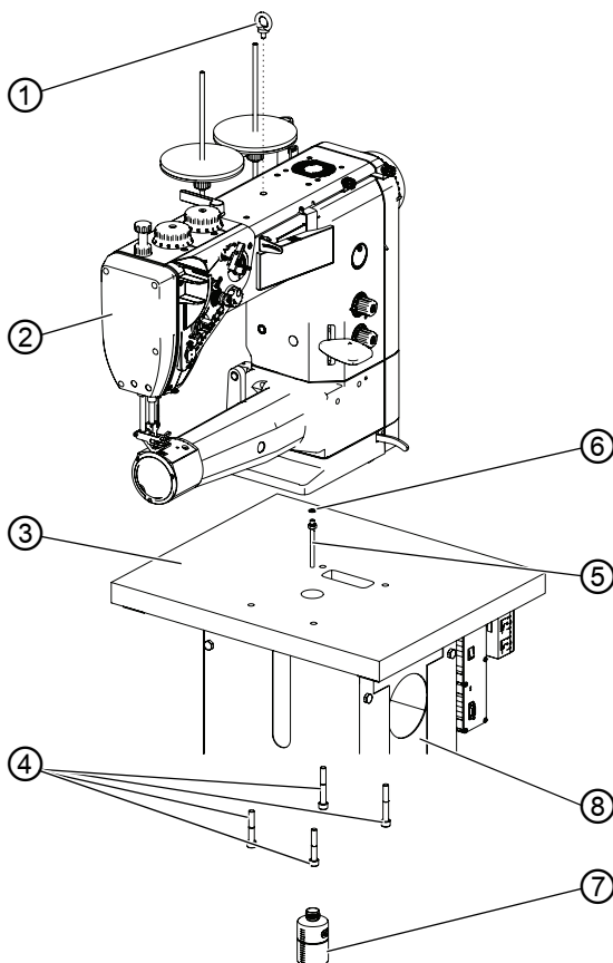
Afb. 60: Bovenste deel van de machine plaatsen (3), wegklapbaar werktafelblad
