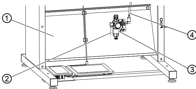
Afb. 65: Onderhoudseenheid voor de perslucht monteren
