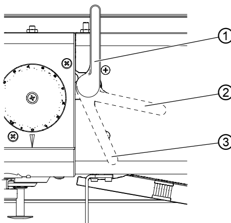
Afb. 26: Naaivoetstand handmatig verhogen
