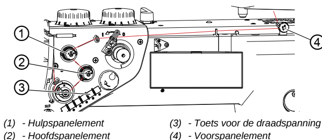
Afb. 18: Bovendraadspanning controleren
