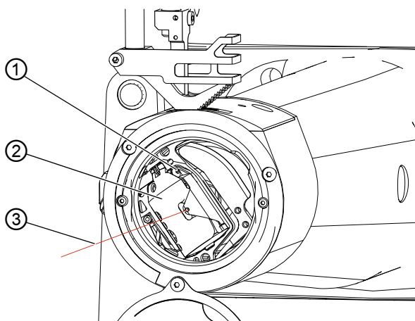
Afb. 19: Onderdraadspanning instellen
