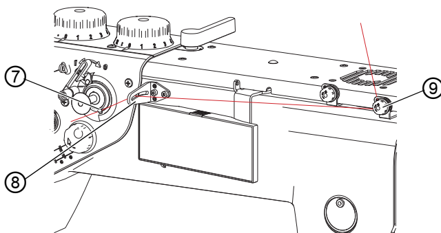
Afb. 11: Onderdraad opwikkelen (2)
