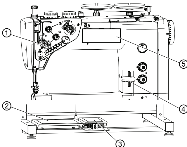
Afb. 32: Achteruitnaaien en afhechting
