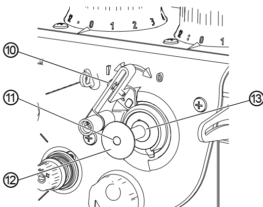
Afb. 12: Onderdraad opwickelen (3)
