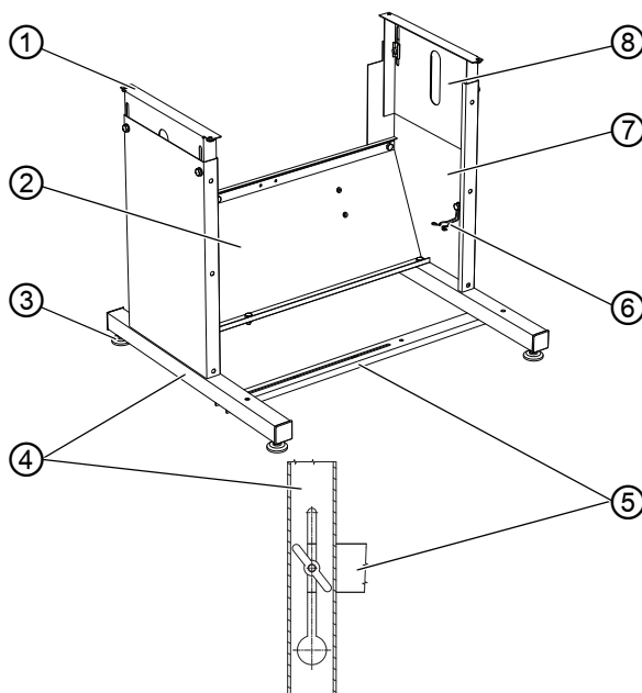
Afb. 47: Onderstel voor machines met een standaardarm monteren
