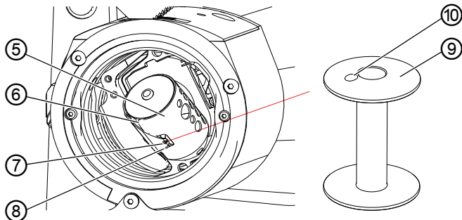
Afb. 15: Spoel vervangen (3)
