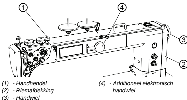
Afb. 22: Machines met een lange arm
