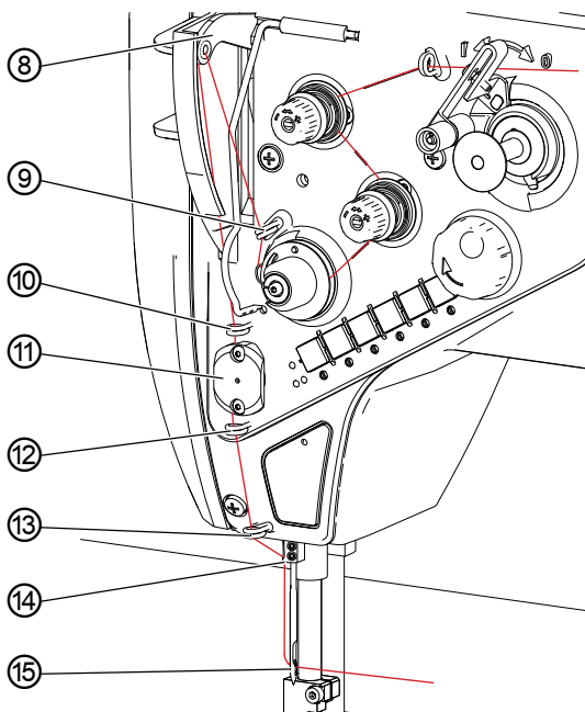
Afb. 9: Bovendraad inrijgen (2)
