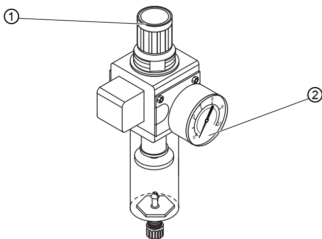
Afb. 44: Werkdruk instellen
