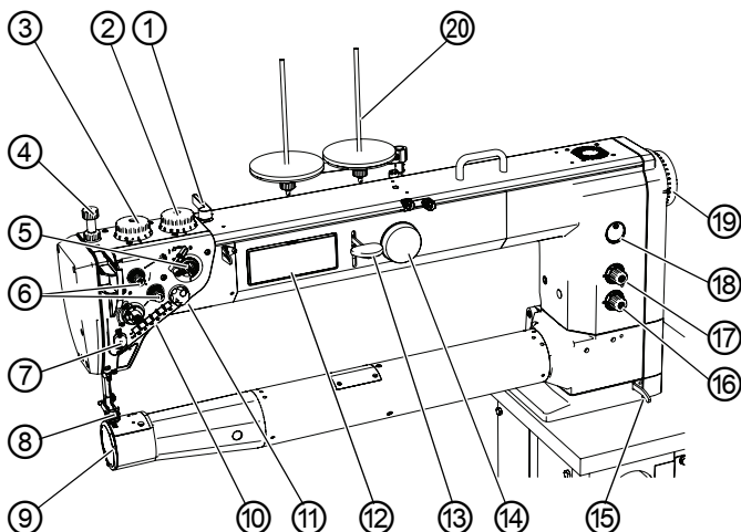
Abb. 3: Componenten van de machine (3), machines met lange arm
