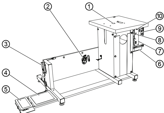
Abb. 4: Componenten van de machine (4), onderstel voor machines met een lange arm
