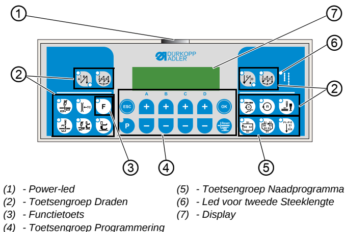
Afb. 41: Programmering
