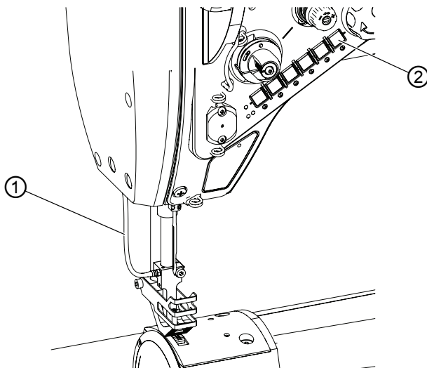
Afb. 38: Naaldkoeling
