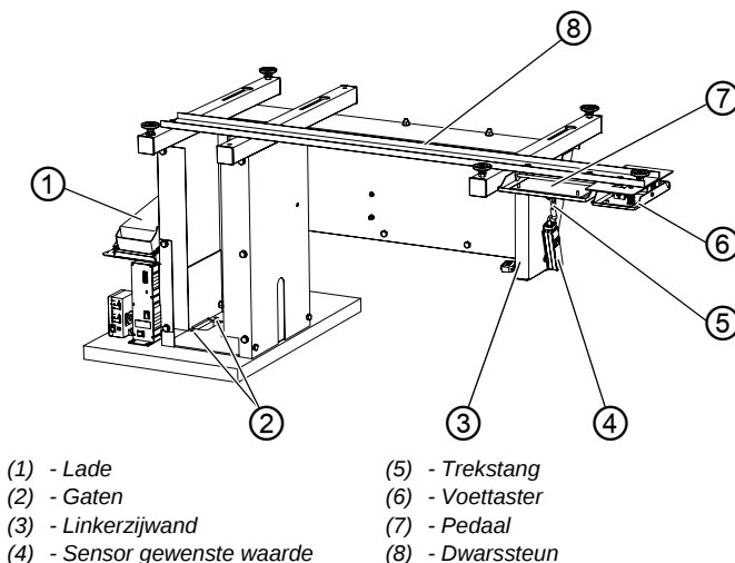
Afb. 54: Werktafelblad voor machines met een lange arm monteren
