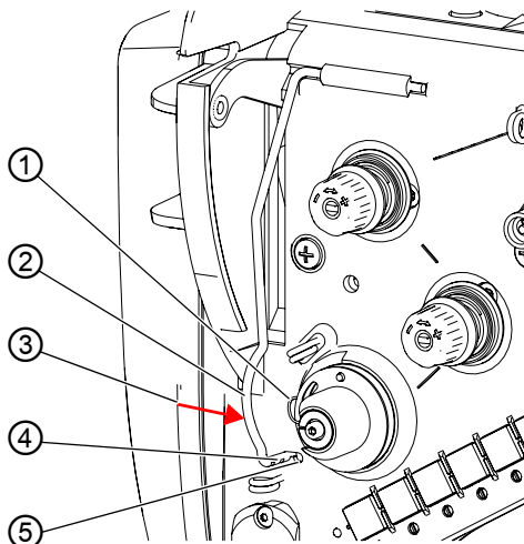
Afb. 20: Bovendraadregelaar instellen
