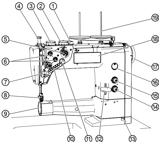
Afb. 1: Componenten van de machine (1), machines met standaardarm
