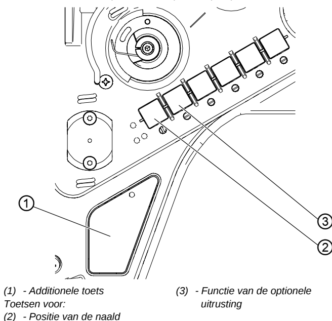
Afb. 34: Snelfuncties op het toetsenpaneel (Eco)
