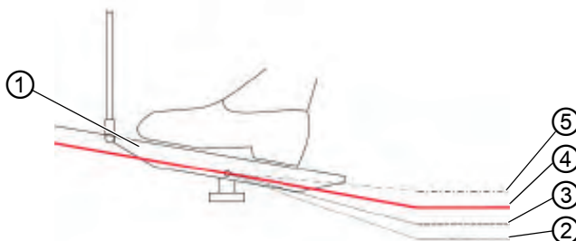
Afb. 25: Naaivoetstand elektropneumatisch verhogen
