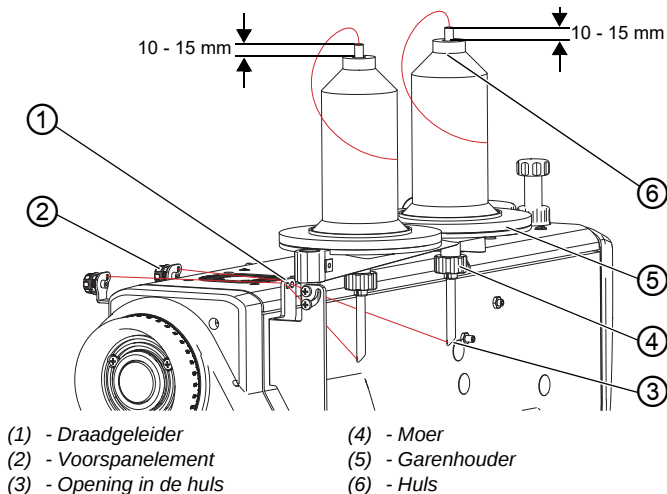
Afb. 7: Bovendraad van de garenklos naar de machine rijgen
