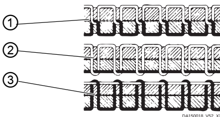
Afb. 16: Draadspanning
