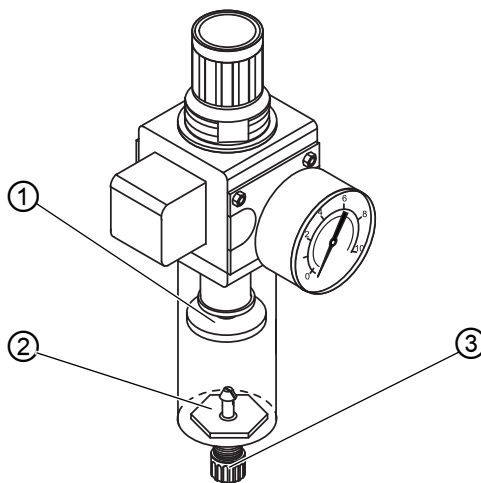
Afb. 46: Filterinzetstuk reinigen
