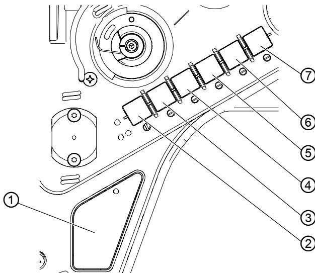
Afb. 33: Snelfuncties op het toetsenpaneel (Classic)
