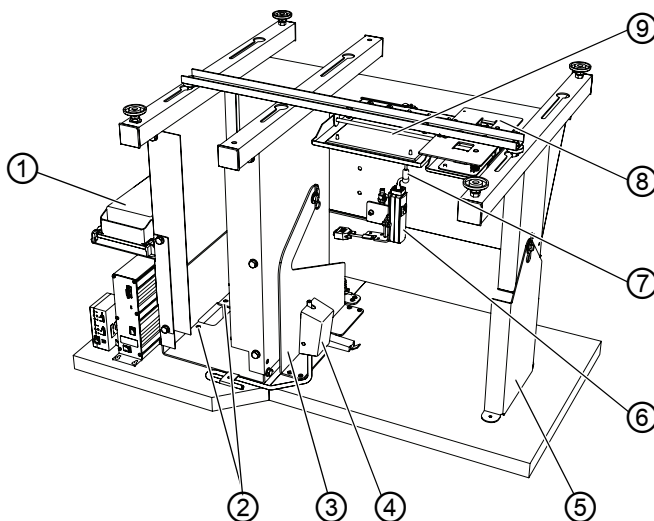
Afb. 55: Wegklapbaar werktafelblad monteren
