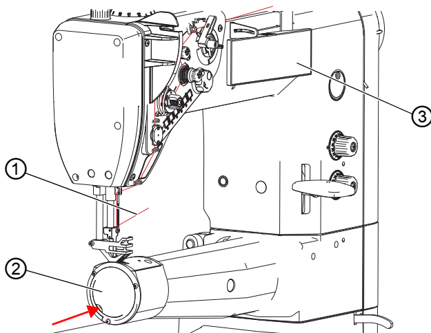
Afb. 13: Spoel vervangen (1)
