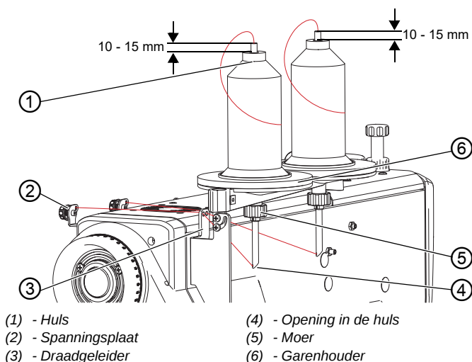
Afb. 10: Onderdraad opwickelen (1)
