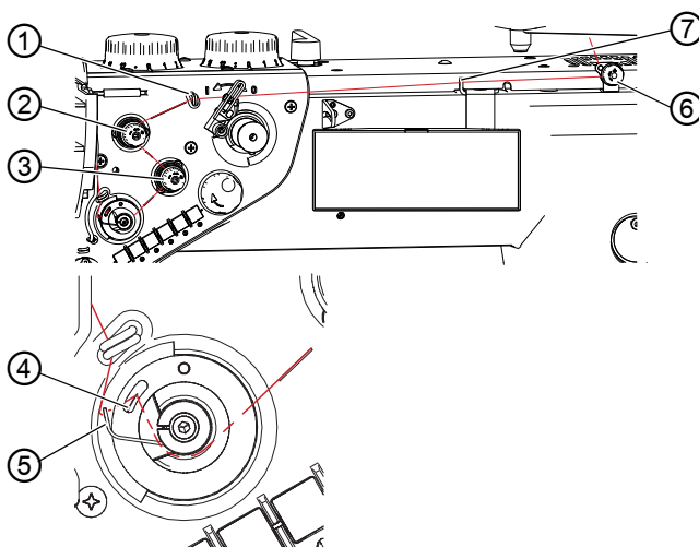
Afb. 8: Bovendraad inrijgen (1)
