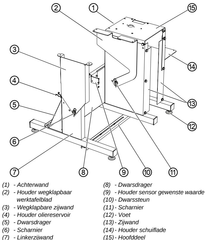
Afb. 49: Wegklapbaar onderstel monteren
