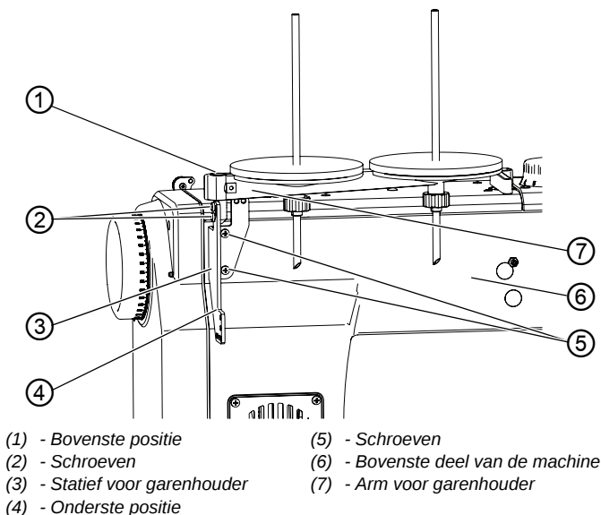
Afb. 61: Garenhouder bevestigen
