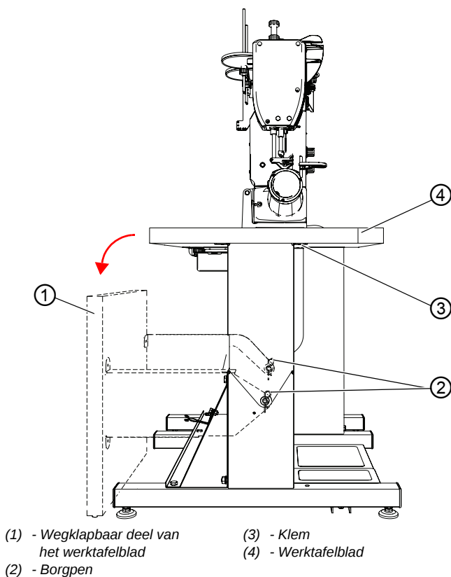
Afb. 39: Werktafelblad omlaag duwen
