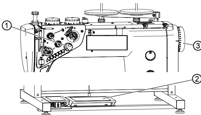
Afb. 24: Naald automatisch positioneren
