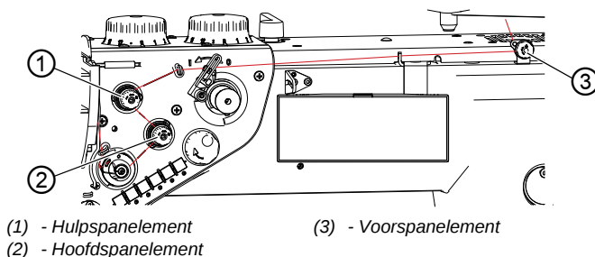
Afb. 17: Bovendraadspanning instellen
