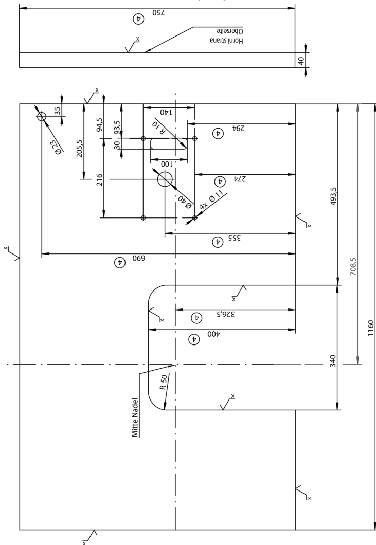
Afb. 67: Vast werktafelblad met uitsparing, machines met een standaardarm
