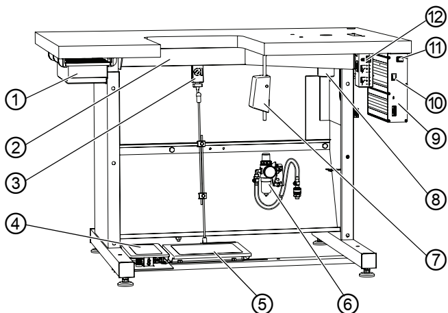
Abb. 2: Componenten van de machine (2), onderstel voor machines met standaardarm
