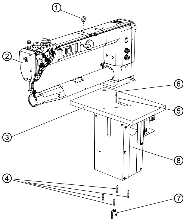
Afb. 59: Bovenste deel van de machine plaatsen (2), machines met lange arm
