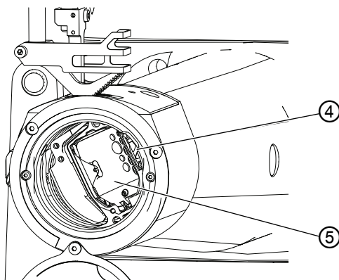
Afb. 14: Spoel vervangen (2)
