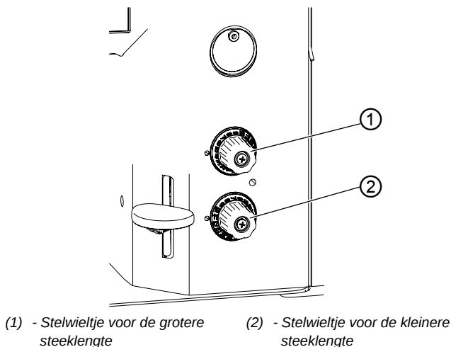
Afb. 30: Steeklengte instellen
