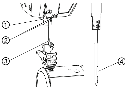
Afb. 6: Naald inzetten of vervangen
