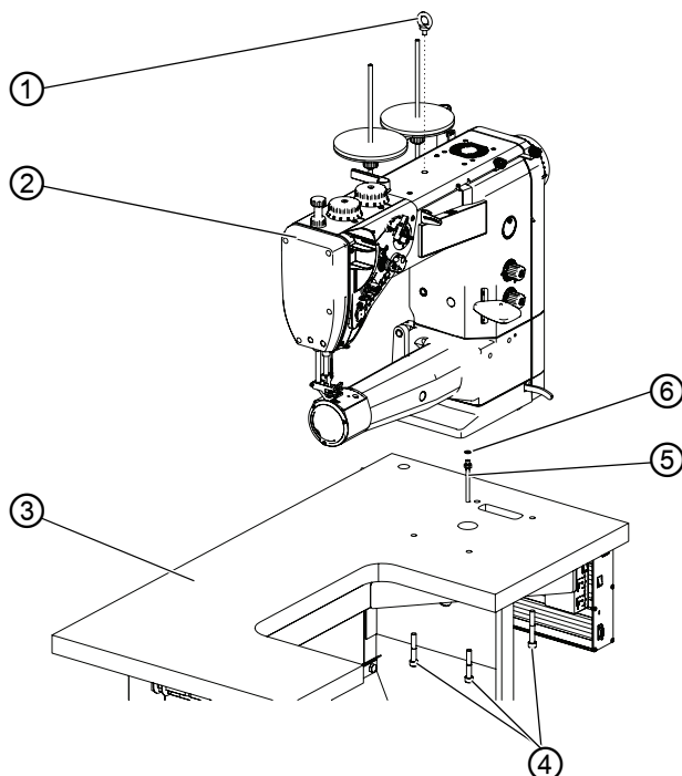
Afb. 58: Bovenste deel van de machine plaatsen (1), machines met standaard arm
