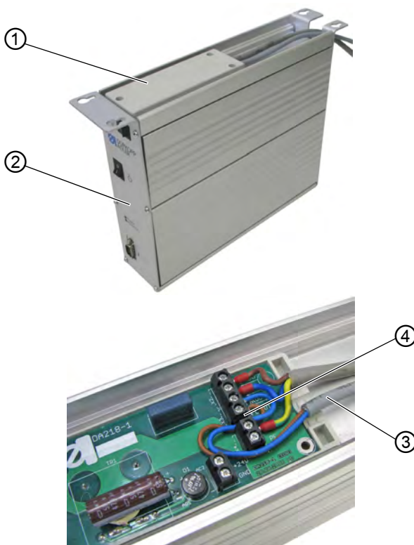
Afb. 62: Naaiverlichting aansluiten (1)
