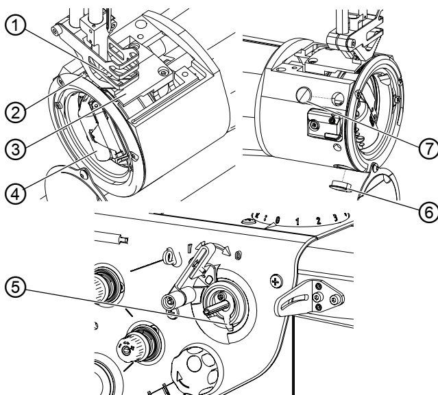
Afb. 42: Reinigen
