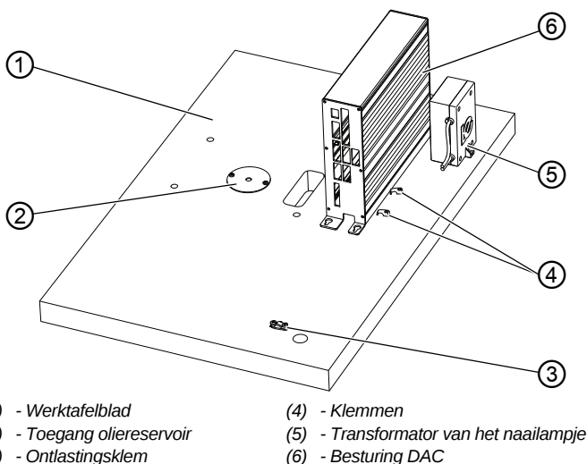
Afb. 51: Machines met een lange arm
