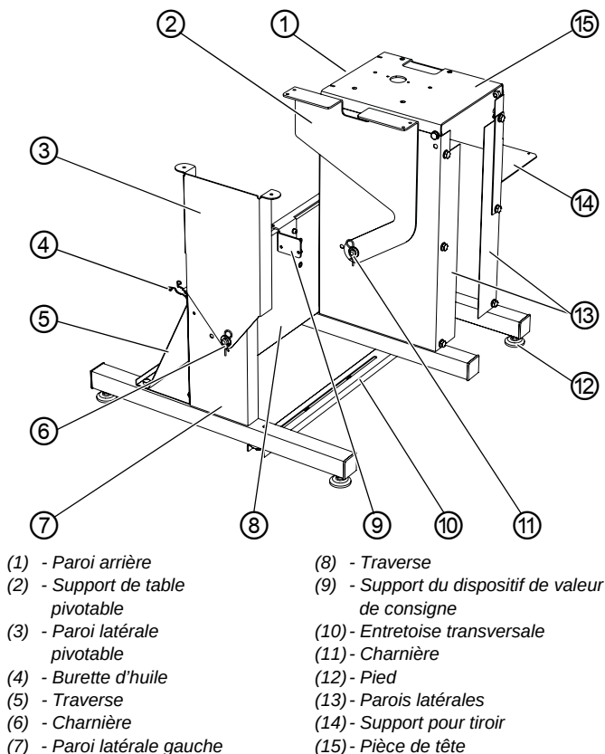
Image 49: Monter le bâti pivotable
