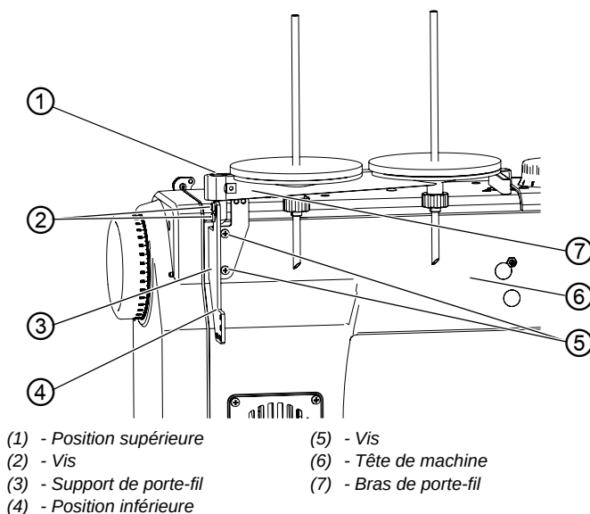
Image 61: Monter le porte-fil
