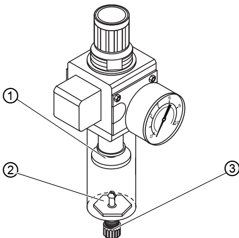
Image 45: Évacuer l'eau de condensation
