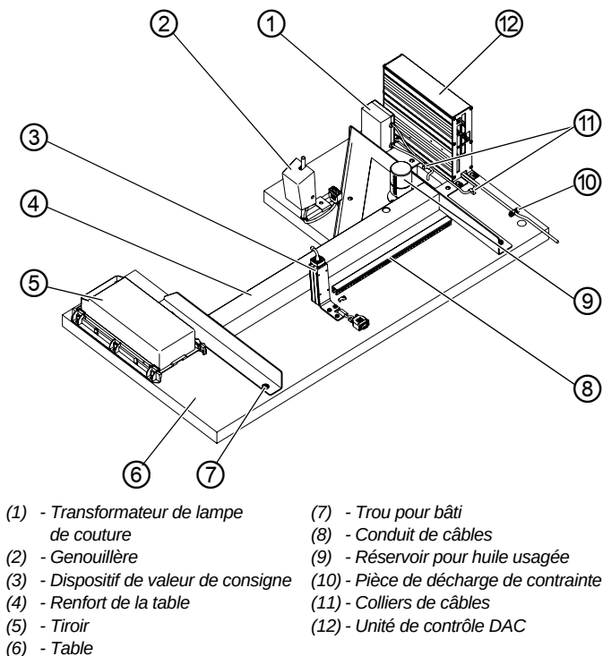
Image 50: Machines à bras standard
