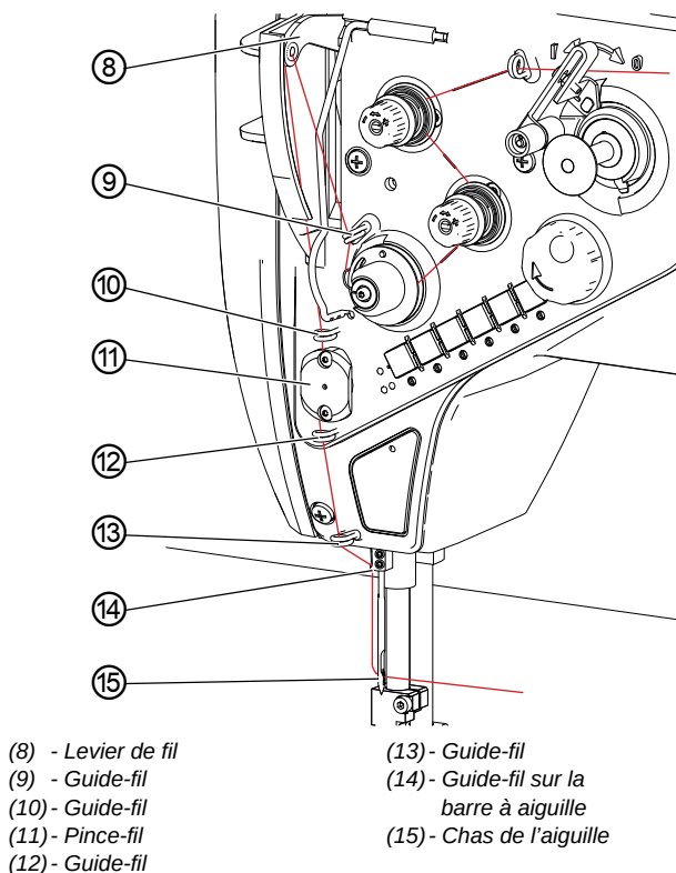
Image 9: Enfiler le fil d'aiguille (2)
