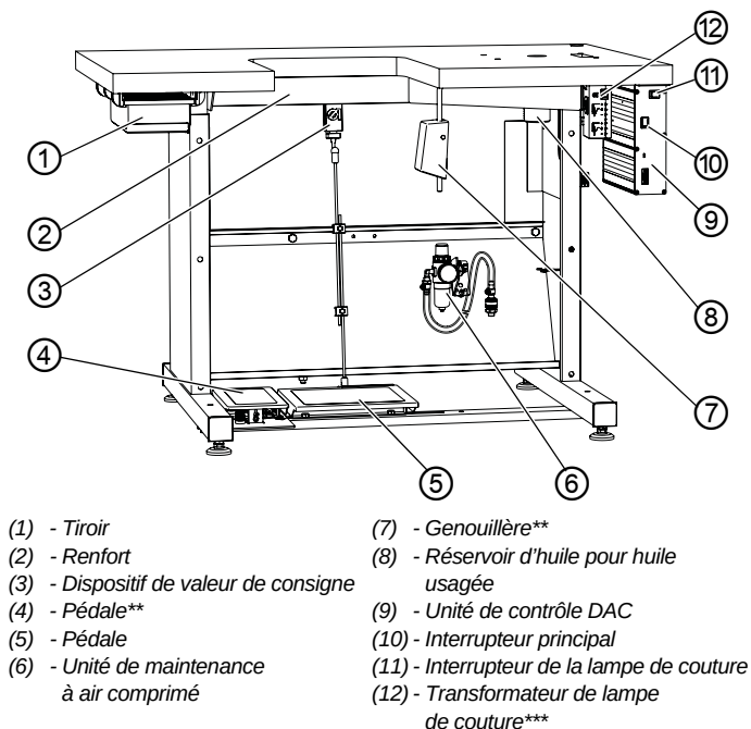
Image 2: Composants de la machine (2), bâti pour les machines à bras standard
