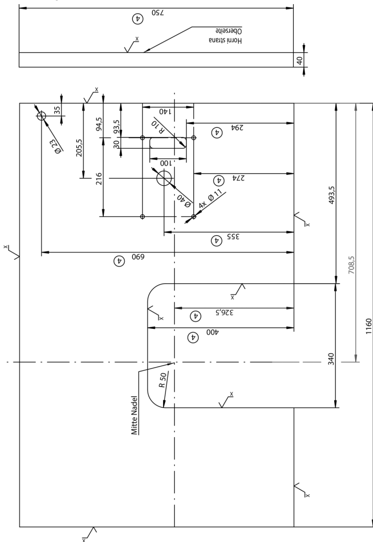
Image 67: Table fixe avec évidemment, machines à bras standard
