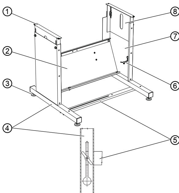
Image 47: Monter le bâti pour machines à bras standard
