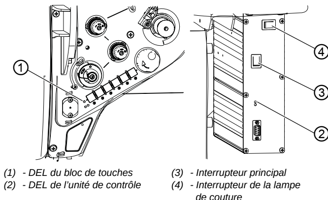
Image 5: Mettre en marche et arrêter la machine
