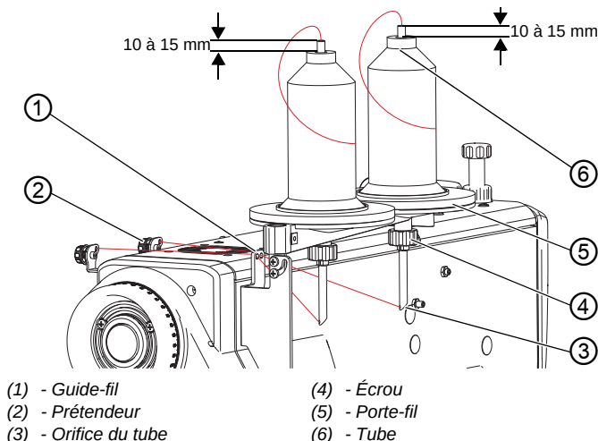
Image 7: Enfiler le fil d'aiguille de la bobine vers la machine
