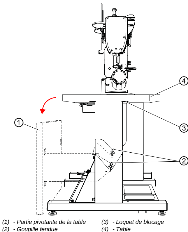
Image 39: Faire pivoter la table vers le bas
