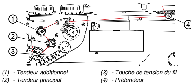
Image 18: Vérifier la tension du fil d'aiguille
