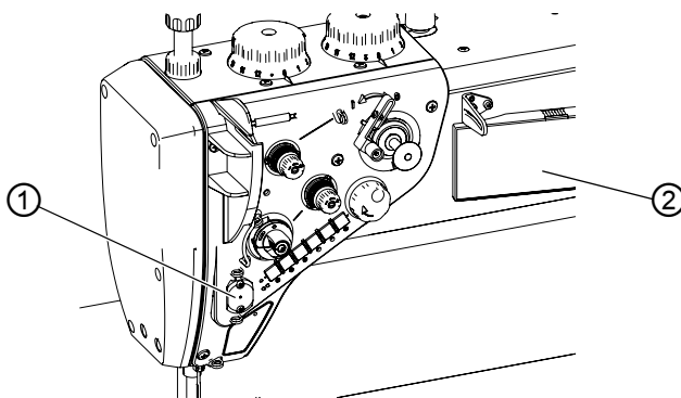
(1) - Pince-fil
