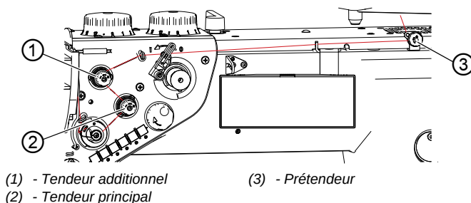
Image 17: Régler la tension du fil d'aiguille
