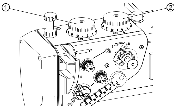
Image 28: Régler la course des pieds presseurs
