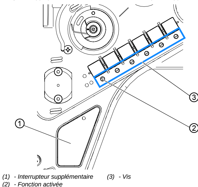
Image 35: Appliquer la fonction des touches à l'interrupteur supplémentaire
