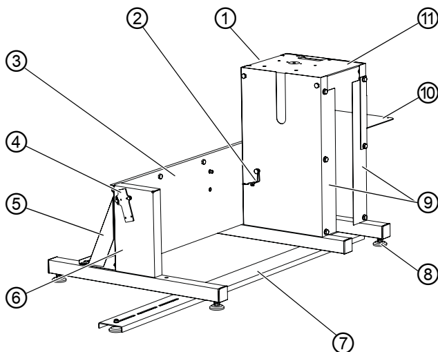
Image 48: Monter le bâti pour machines à bras long
