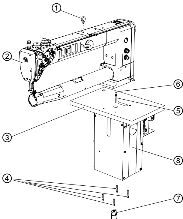
Image 59: Insérer la tête de machine (2), machines à bras long
