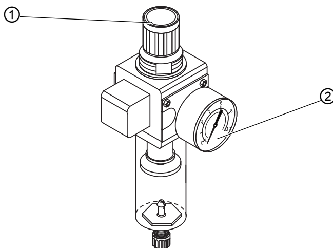
Image 66: Régler la pression de service
