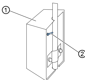
Image 29: Régler le réglage rapide de la course à l'aide de la genouillère
