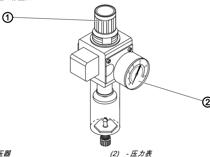
图 72: 设置工作压力
