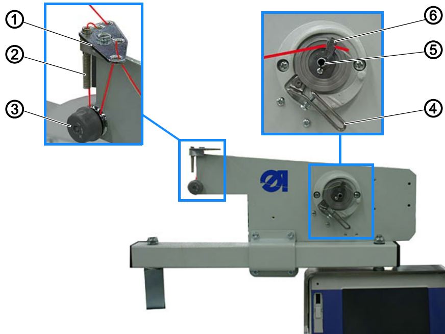
图 8: 绕梭芯线
