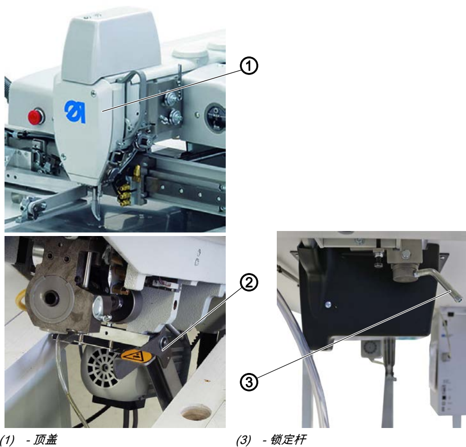
图 14: 转回机头
