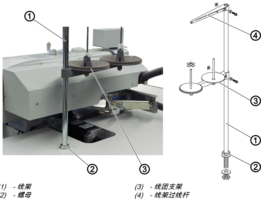
图 67: 安装线架
