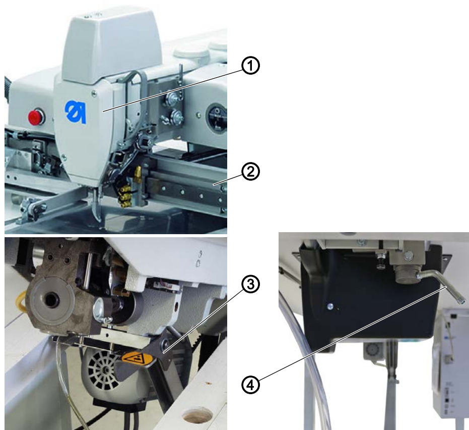
图 13: 竖起机头
