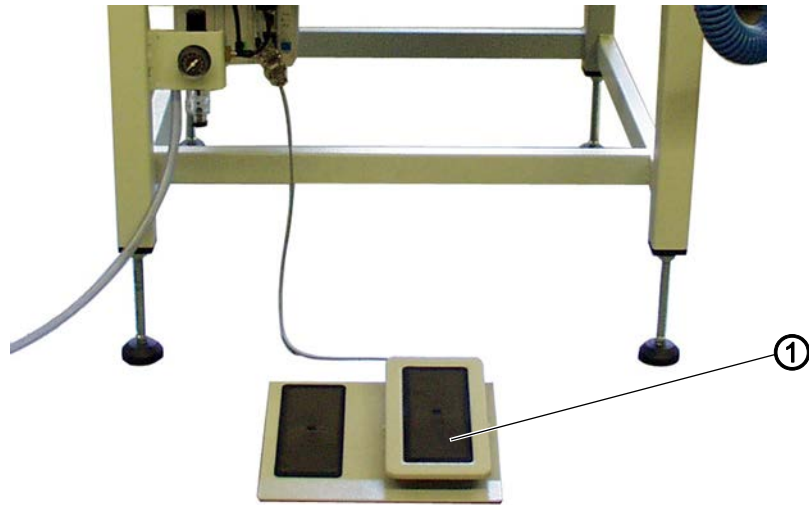
图 66: 调整踏板
