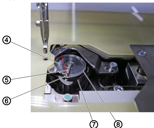
图 10: 更换梭芯 (2)
