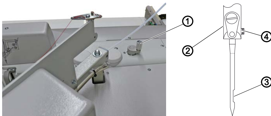
图 4: 更换机针
