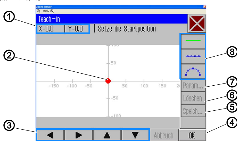
图 35: 新建线缝程序
