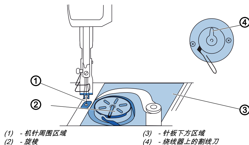
图 56: 清洁机器
