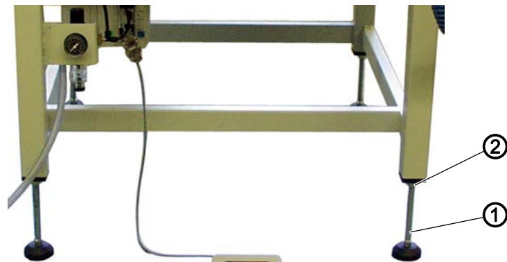
图 65: 设置不带滚轮的机架的工作高度
