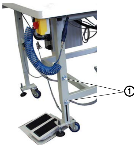
图 64: 设置带滚轮的机架的工作高度
