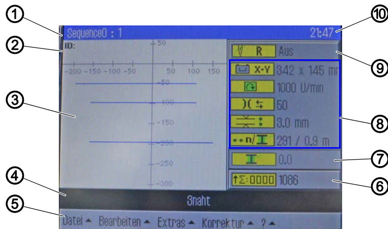
图 17: 主屏幕
