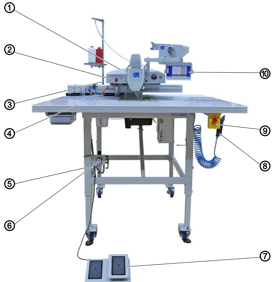
图 1: 机器组件
