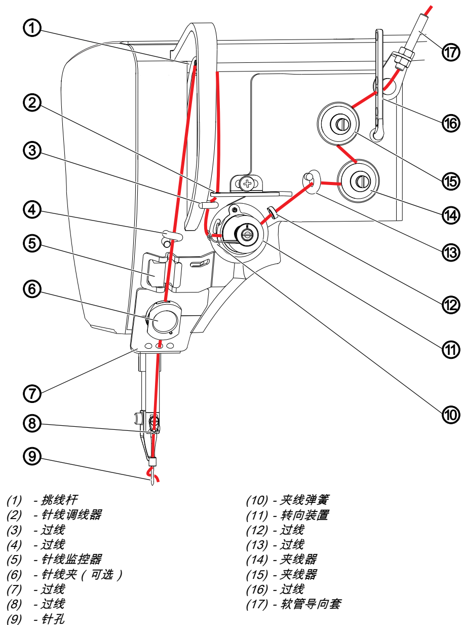
图 6: 穿针线
