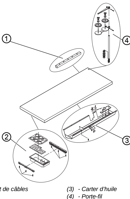
Image 61: Compléter la table
