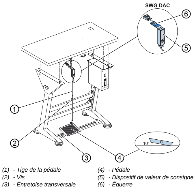
Image 60: Montage de la pédale du dispositif de valeur de consigne
