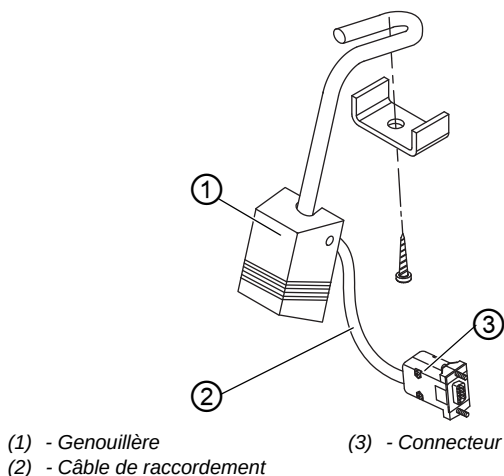
Image 67: Monter la genouillère
