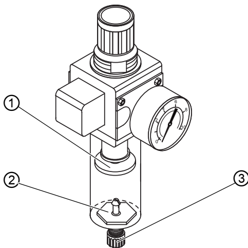
Image 57: Évacuer l'eau de condensation
