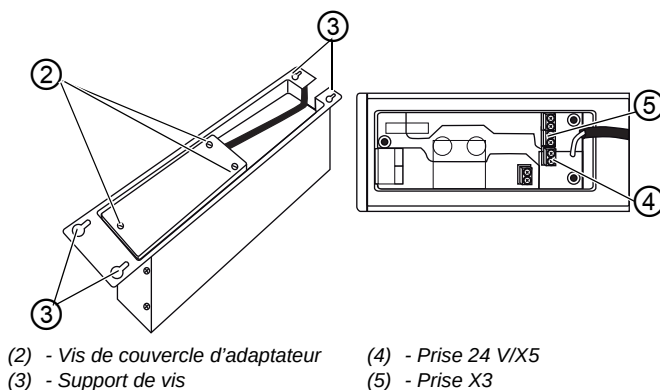
Image 69: Raccorder le transformateur de lampe de couture (2)
