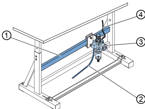
Image 71: Monter l'unité de maintenance à air comprimé
