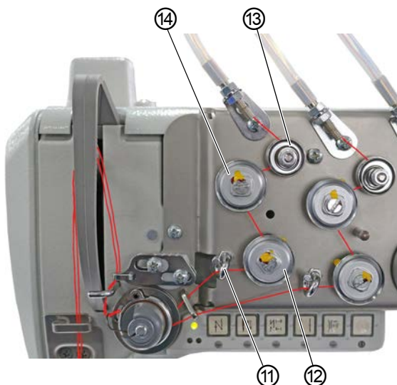
Image 12: Enfiler le fil d'aiguille (machine à 2 aiguilles) (3)
