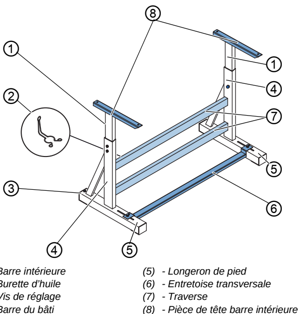
Image 59: Montage du bâti
