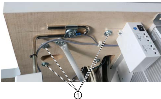
Image 65: Installer la tête de machine (1)
