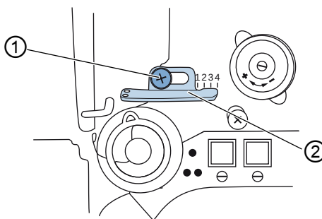
Image 23: Régler le régulateur de fil d'aiguille
