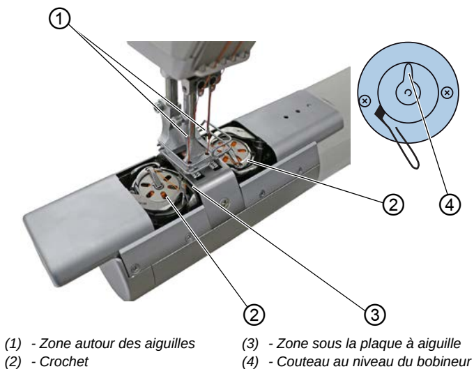
Image 53: Endroits dont le nettoyage est particulièrement important
