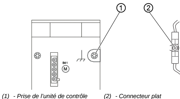
Image 70: Établir la liaison équipotentielle
