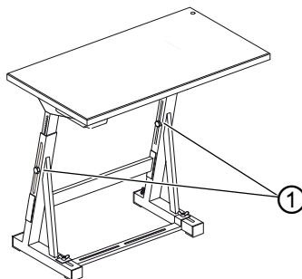
Image 63: Régler la hauteur de travail
