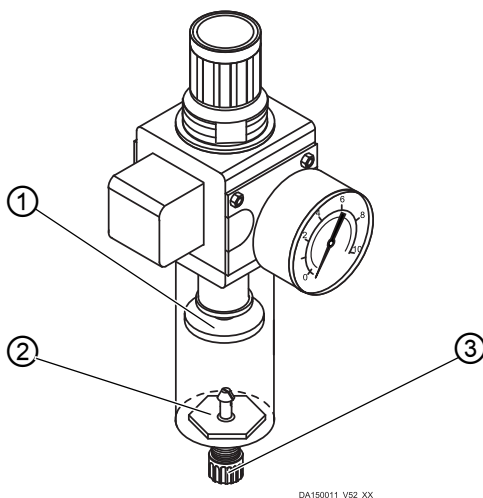
Image 58: Nettoyer l'élément filtrant
