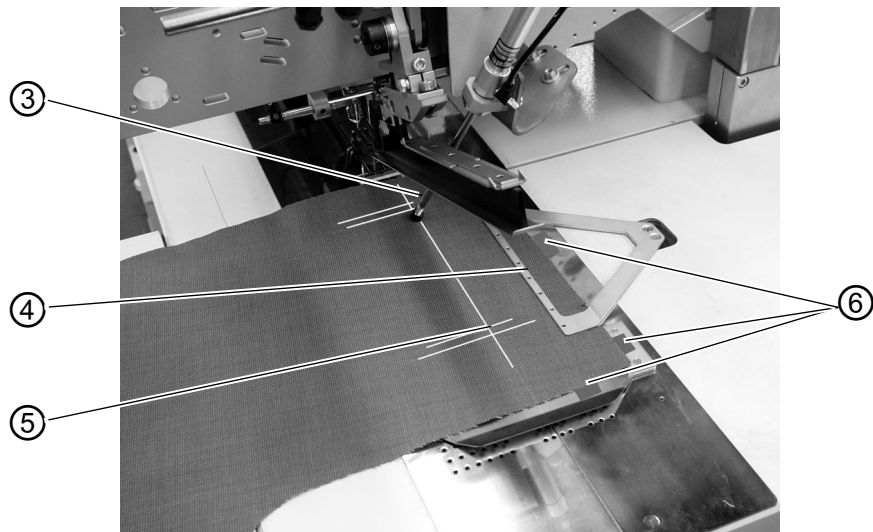
Abb. 33: 2. Schritt Methode A
