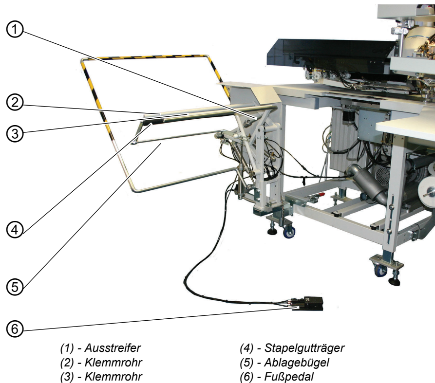
Abb. 52: Überwurfstapler ausgeschwenkt
