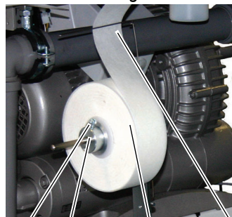
Abb. 56: Bandzuführung
