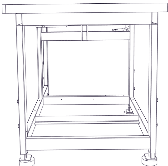
Abb. 66: Nähanlage mit Gestell ohne Rollen
