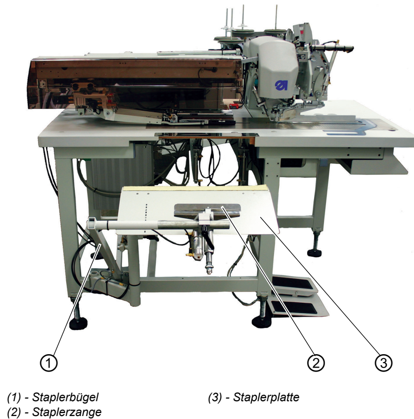
Abb. 50: Zangenstapler
