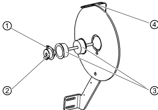
Abb. 57: Bandzuführung im Detail (ohne Bandrolle dargestellt)
