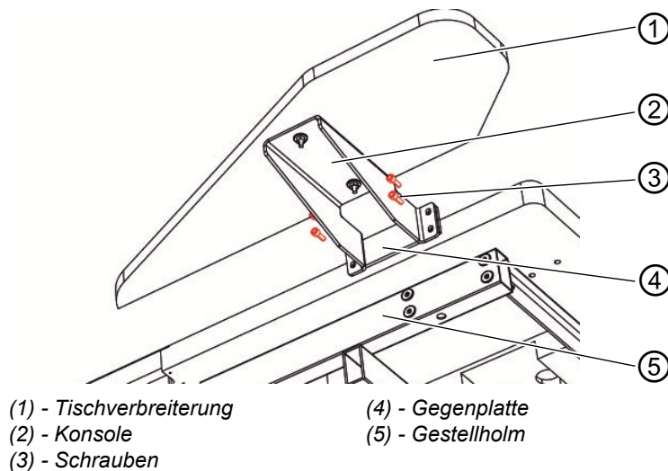
Abb. 75: Tischverbreiterung
