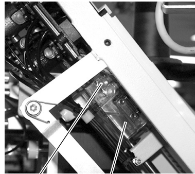
Abb. 65: Ölvorratsbehälter Greiferschmierung
