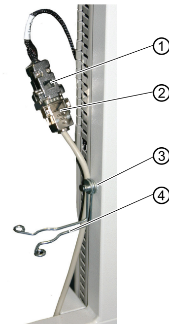
Abb. 69: Anschluss Fußpedal
