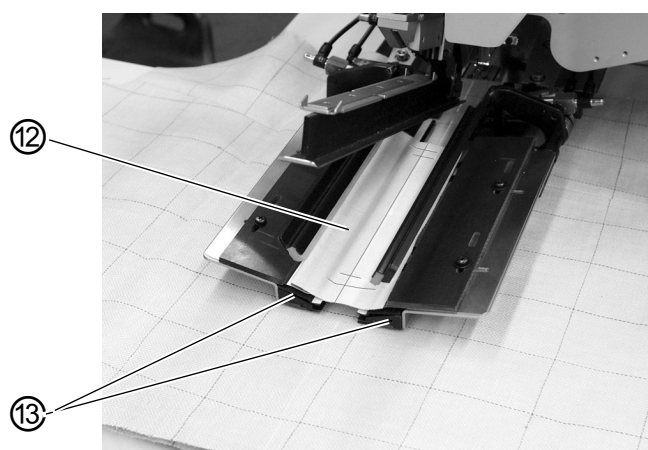
Abb. 44: Anlegehilfe
