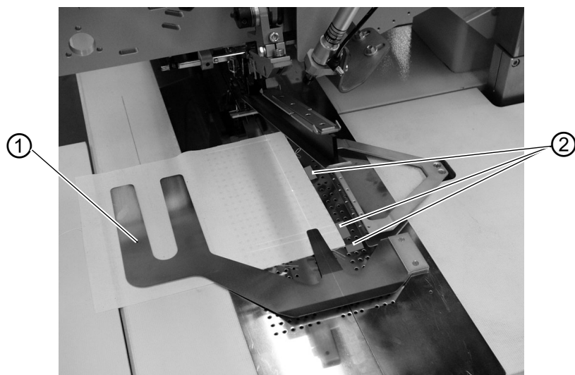
(1) - Taschenbeutelklemme
