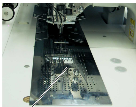
Abb. 81: Anschluss Vakuumanlage
