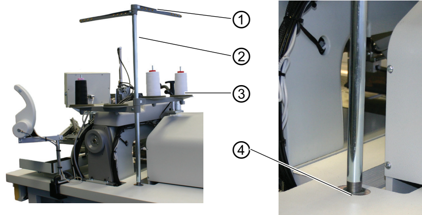
Abb. 71: Garnständer befestigen
