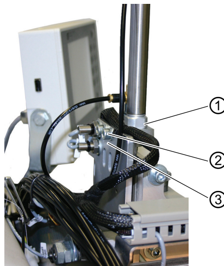
Abb. 72: Zylinder anbringen
