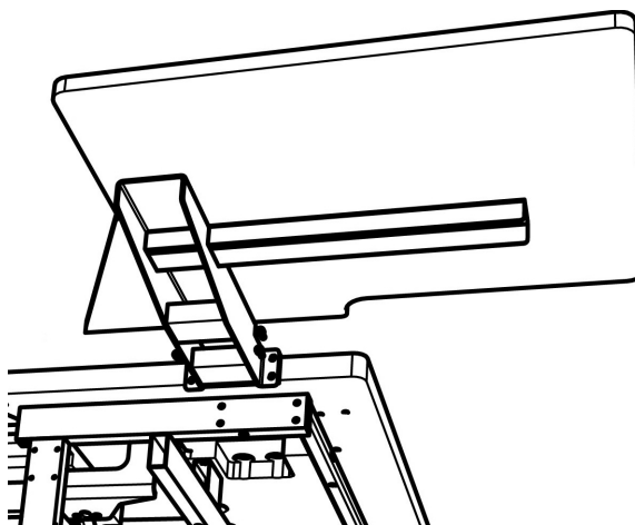
Abb. 76: Tischverbreiterung zum Abstapeln
