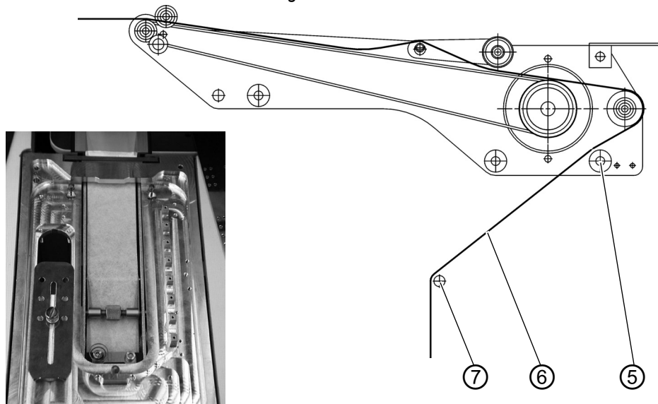
Abb. 59: Funktionsweise Bandzuführung
