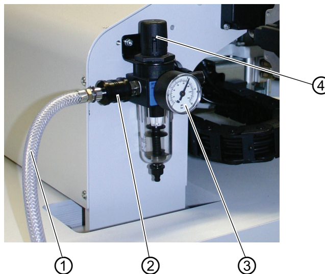
Abb. 80: Pneumatischer Anschluss
