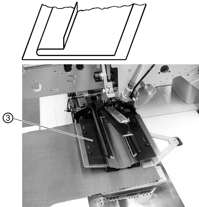
Abb. 37: Einfachpaspel links
