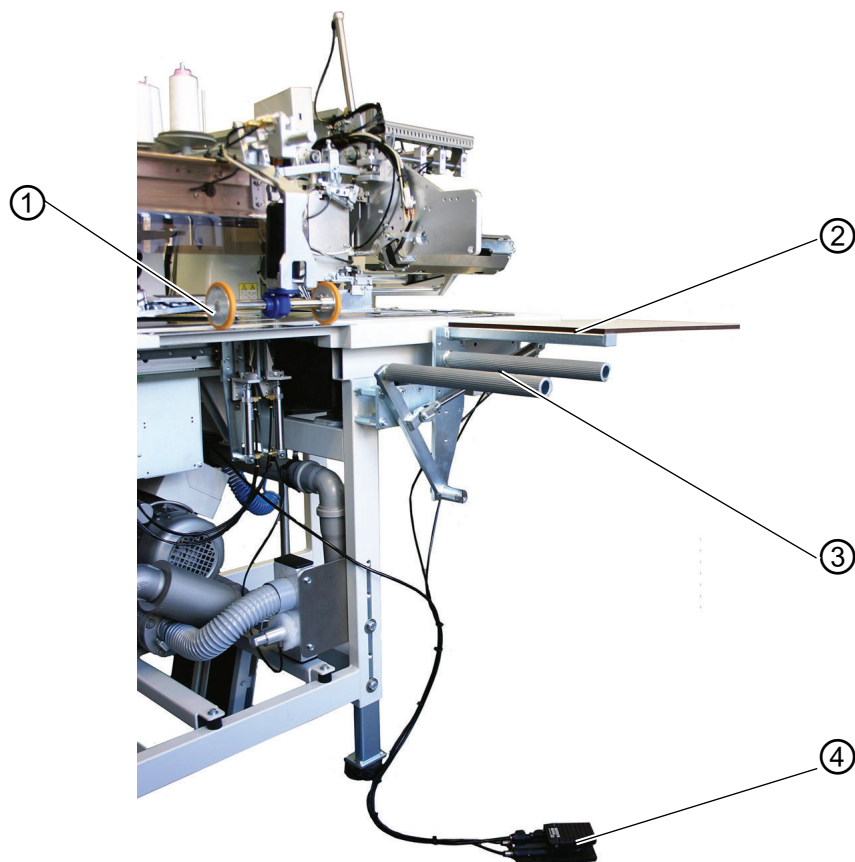
Abb. 55: Bündelklemme
