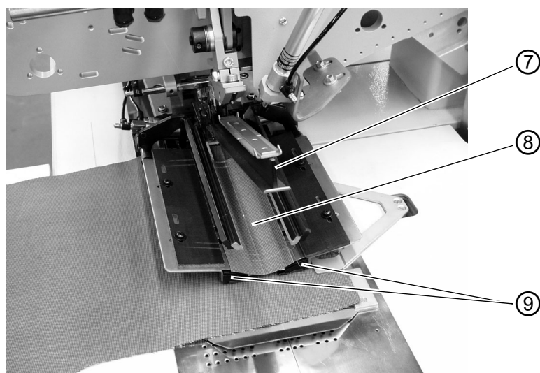
Abb. 34: 3. Schritt Methode A
