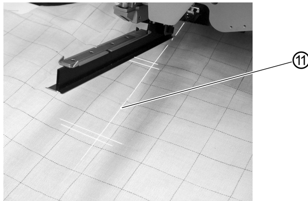
(11) - Tascheneinschnitt
