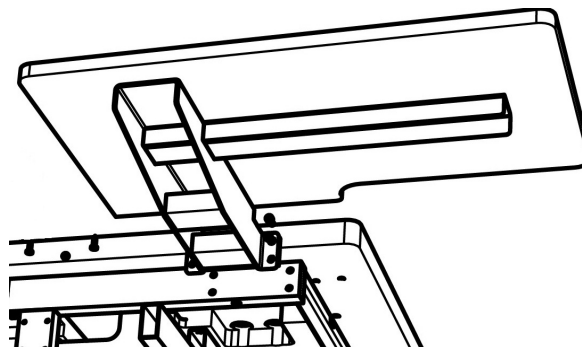
Abb. 77: Anbringung Tischverbreiterung
