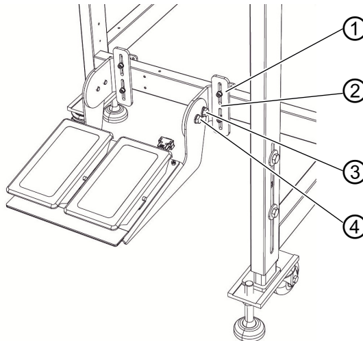
Abb. 70: Fußpedal bei höhenverstellbarem Gestell
