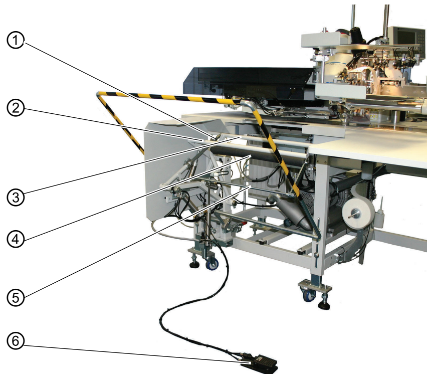
Abb. 51: Überwurfstapler arretiert
