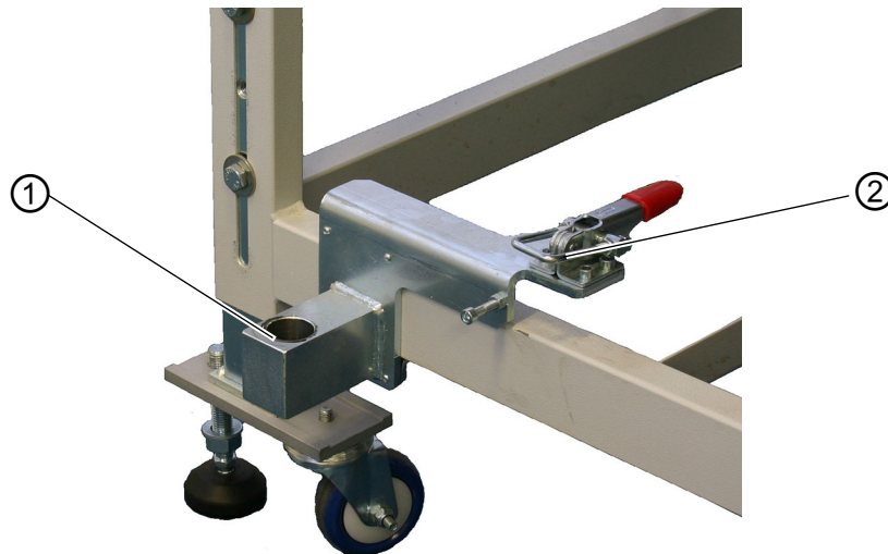
Abb. 49: Aufnahme des Staplers
