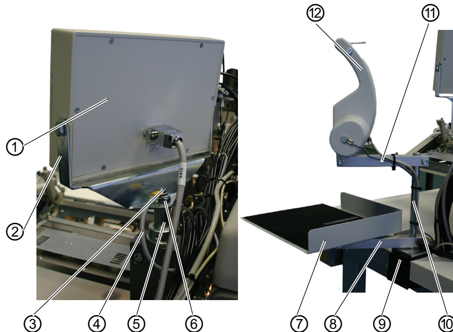
Abb. 74: Haltevorrichtung
