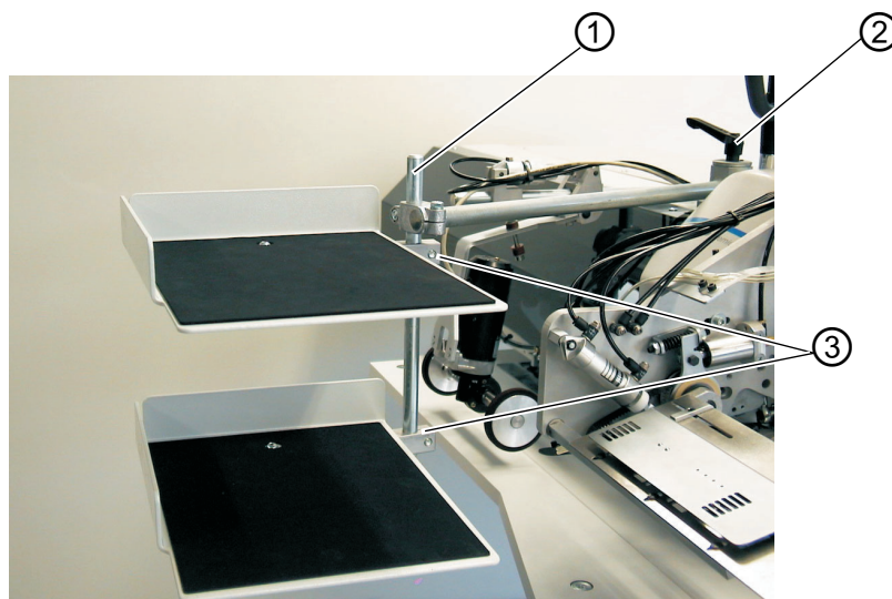
Abb. 73: Vorlagekästen
