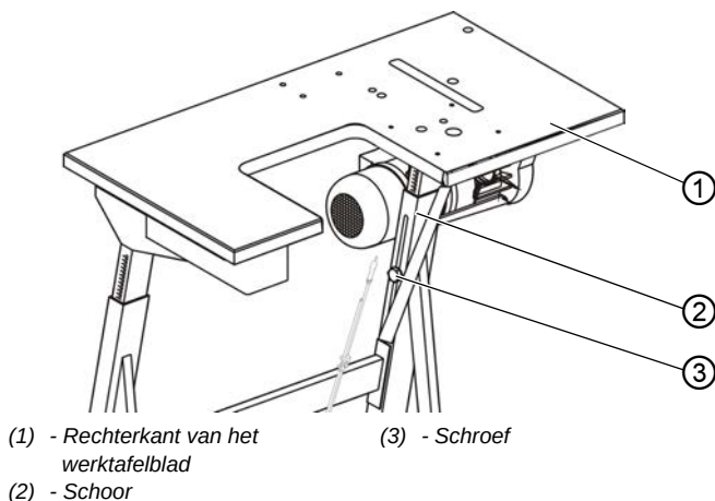
Afb. 42: De steunen monteren bij het werktafelblad met uitsparing
