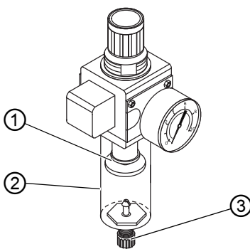
Afb. 30: Filterinzetstuk reinigen
