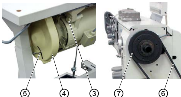
Afb. 51: Riem leggen en spannen (2)
