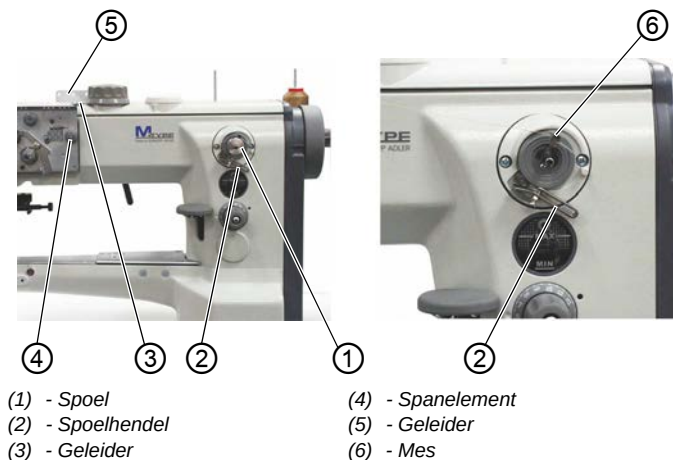
Afb. 5: Onderdraad opwickelen
