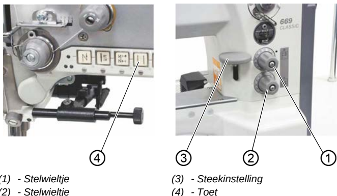
Afb. 18: Steeklengte instellen
