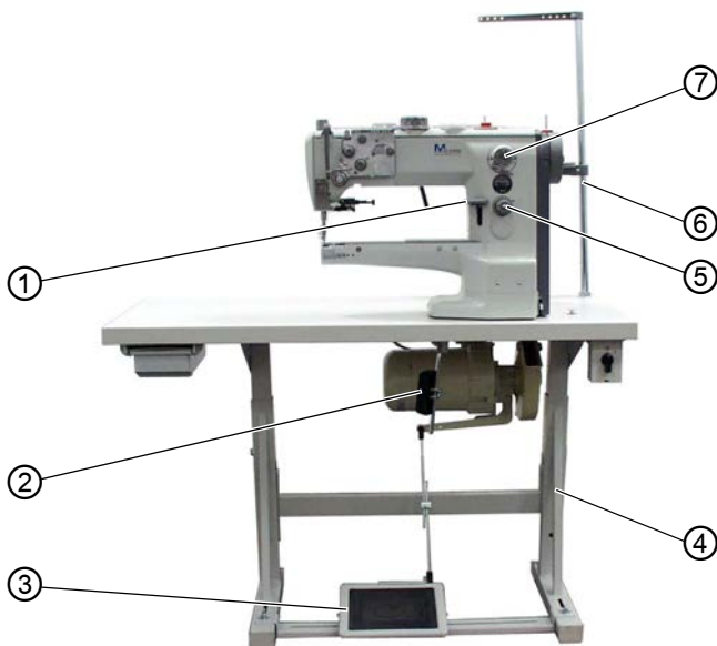
Afb. 1: Componenten van de machine (1), met onderstel MG 55-3
