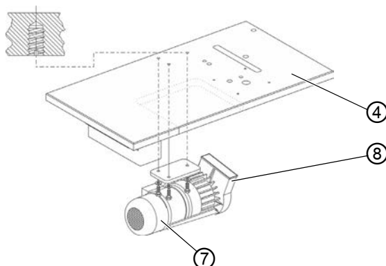
Afb. 35: Werktafelblad opstellen (2)
