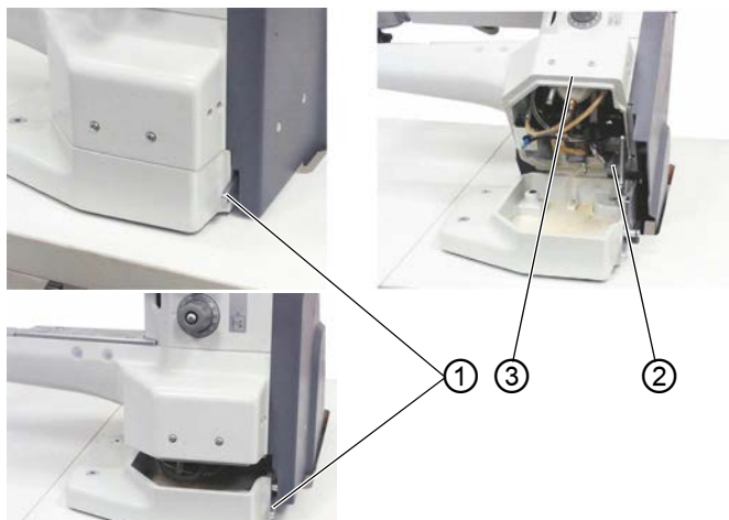
Afb. 20: Bovenste deel naar beneden klappen
