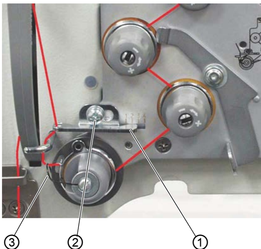
Afb. 12: Draadregelaar instellen
