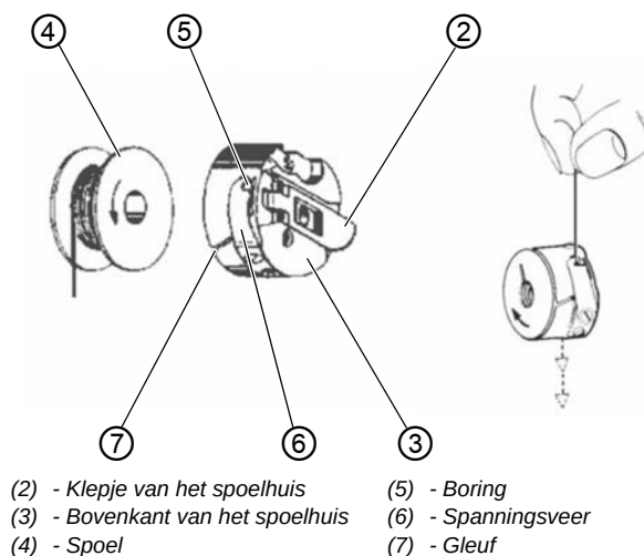
Afb. 7: Onderdraadspoel vervangen (2)
