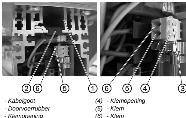
Afb. 64: Naailampje aansluiten
