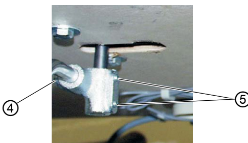
Afb. 53: Kniehendel instellen (2)
