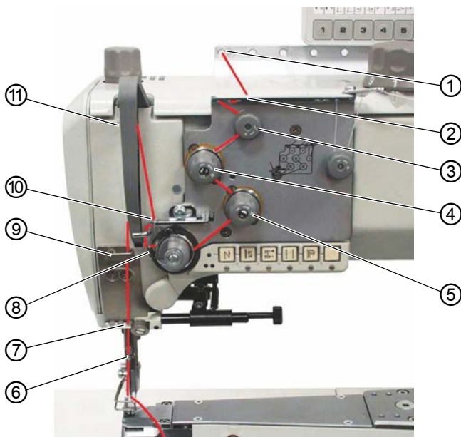
Afb. 4: Bovendraad inrijgen
