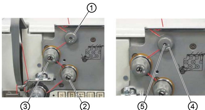
Afb. 9: Bovendraadspanning instellen
