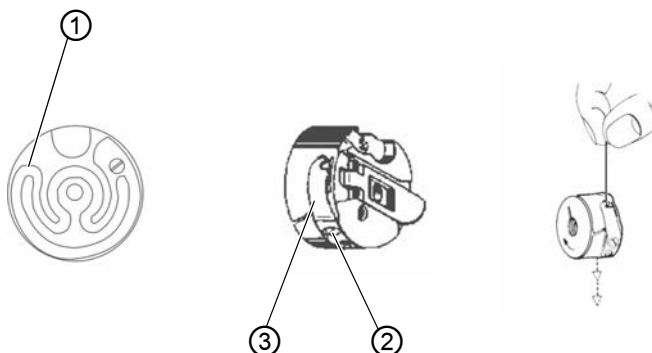
Afb. 11: Onderdraadspanning instellen
