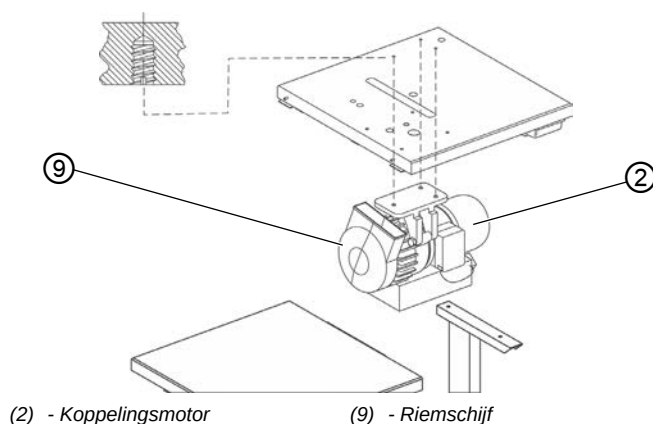
Afb. 38: Werktafelblad opstellen (2)
