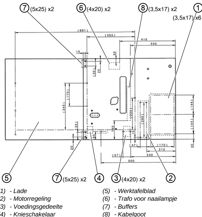
Afb. 39: Werktafelblad opstellen
