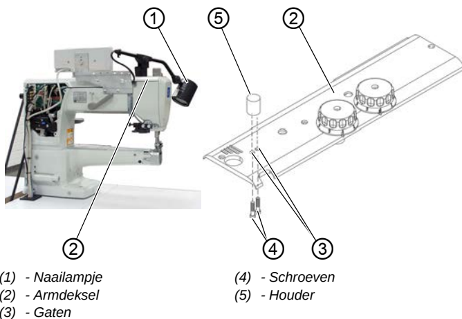
Afb. 46: Naailampje monteren (1)
