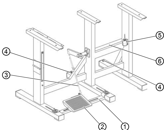
Afb. 33: Onderstel MG 56-3 monteren
