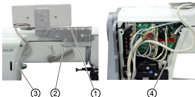
Afb. 45: Bedieningspaneel monteren
