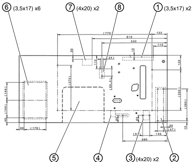
Afb. 36: Werktafelblad opstellen
