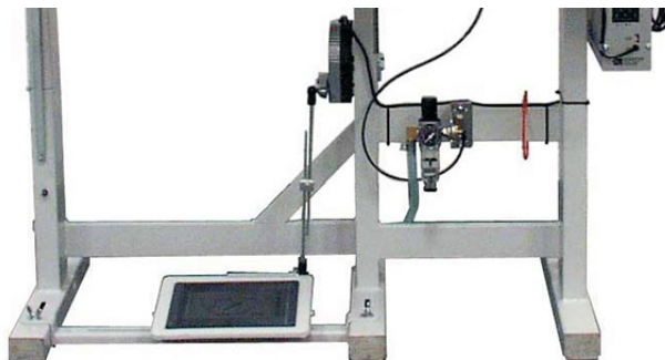
Afb. 65: Onderhoudseenheid voor de perslucht monteren
