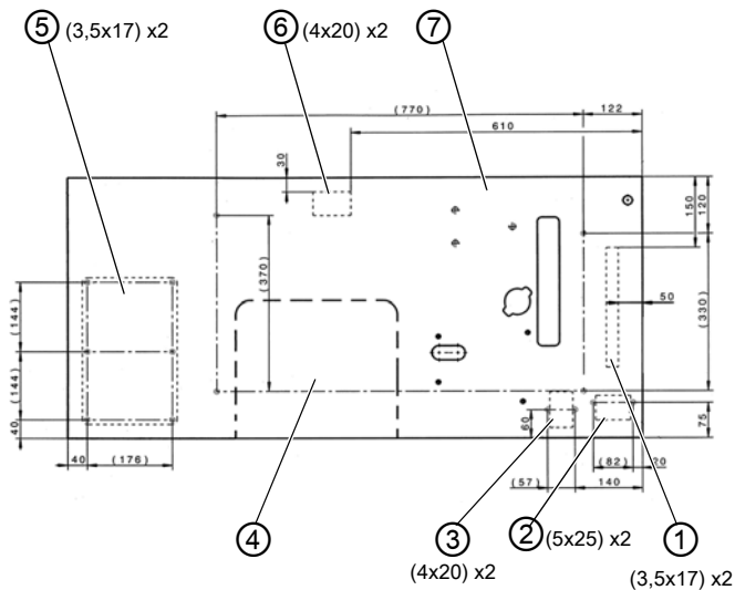
Afb. 34: Werktafelblad opstellen (1)
