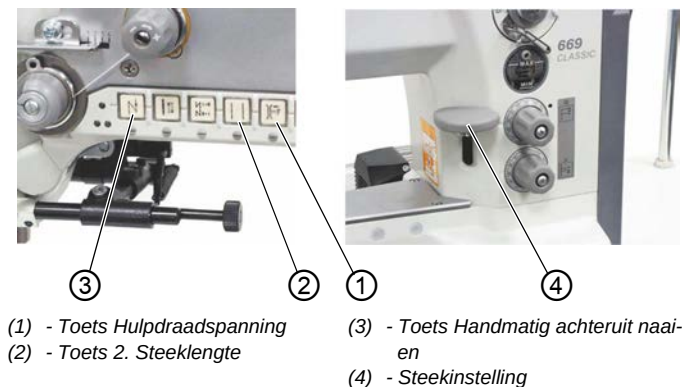
Afb. 25: Naaïen met machines met positioneeraandrijving Efka (2)
