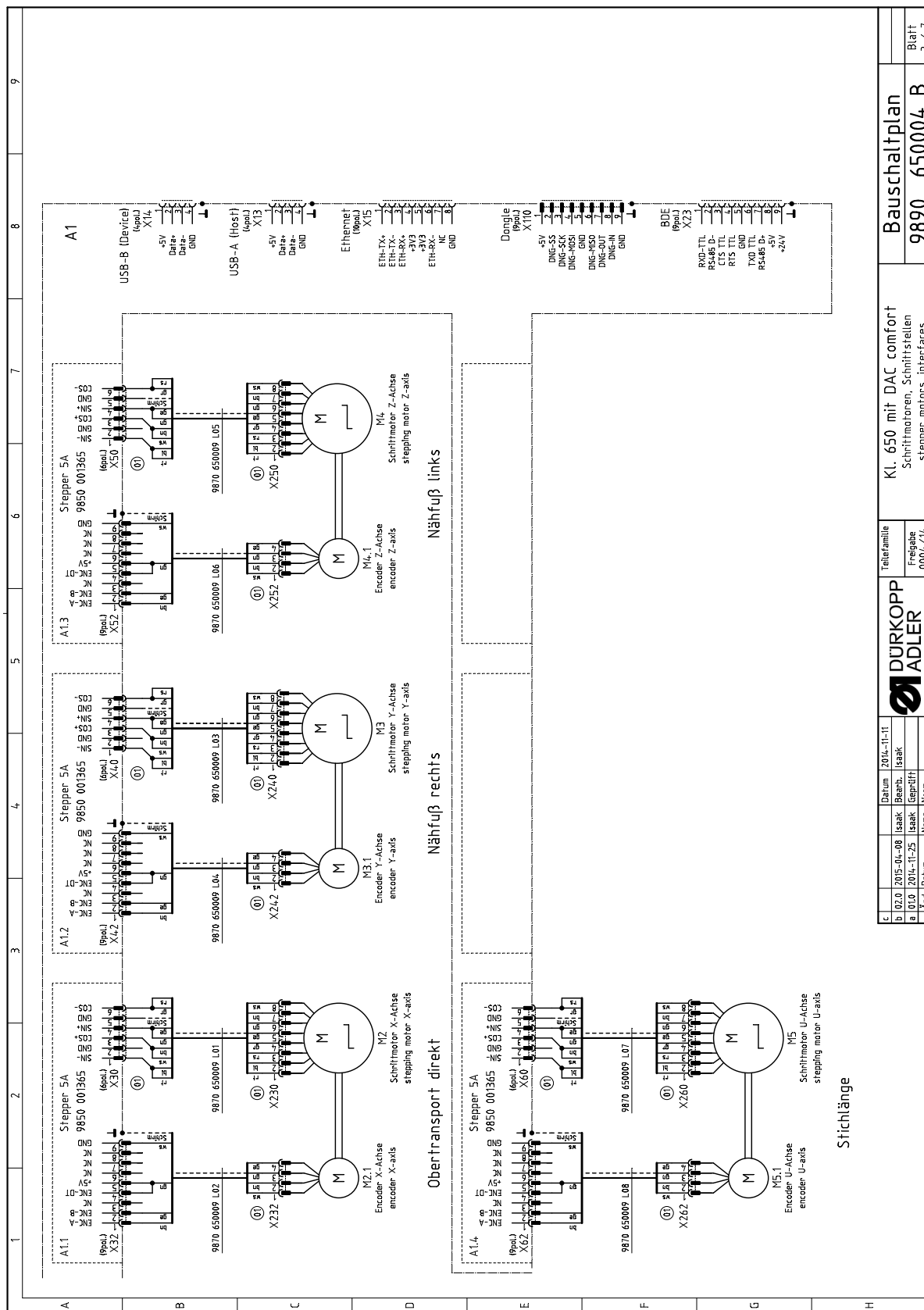
图 91: 接线图
