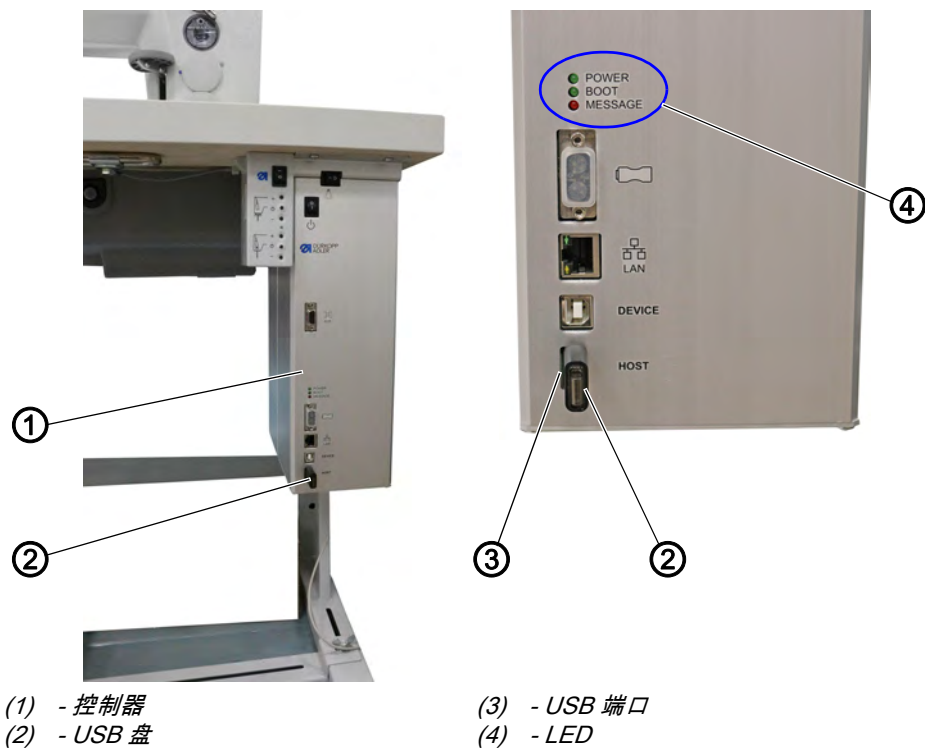
图 68: 执行软件升级 (1)
