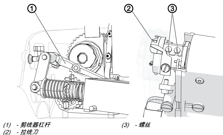
图 17: 更换和设置拉线刀
