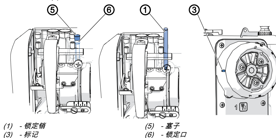
图 8: 锁定机器 (2)
