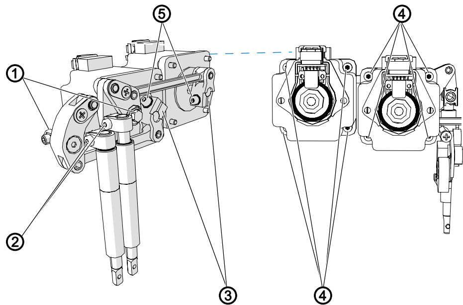
图 32: 检查缝纫压脚提升传动装置
