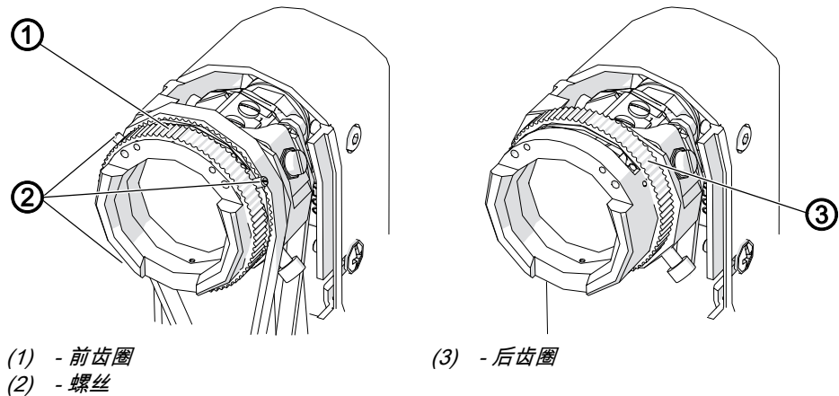
图 31: 更换齿圈
