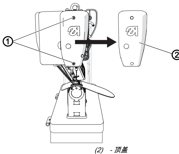
图 2: 拆卸和安装顶盖
