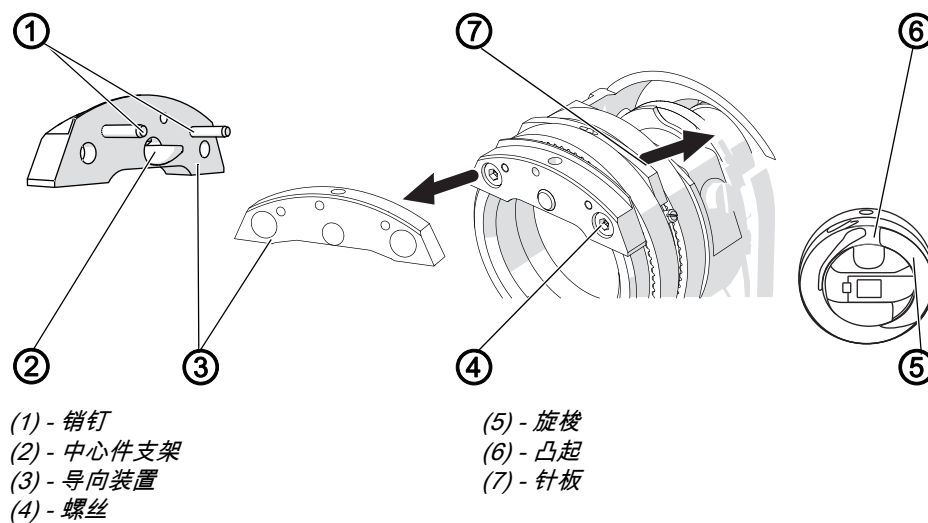
图 5: 拆卸和安装针板
