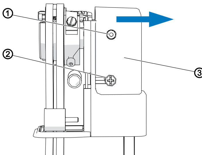
图 23: 设置旋梭驱动装置的齿形带 (1)
