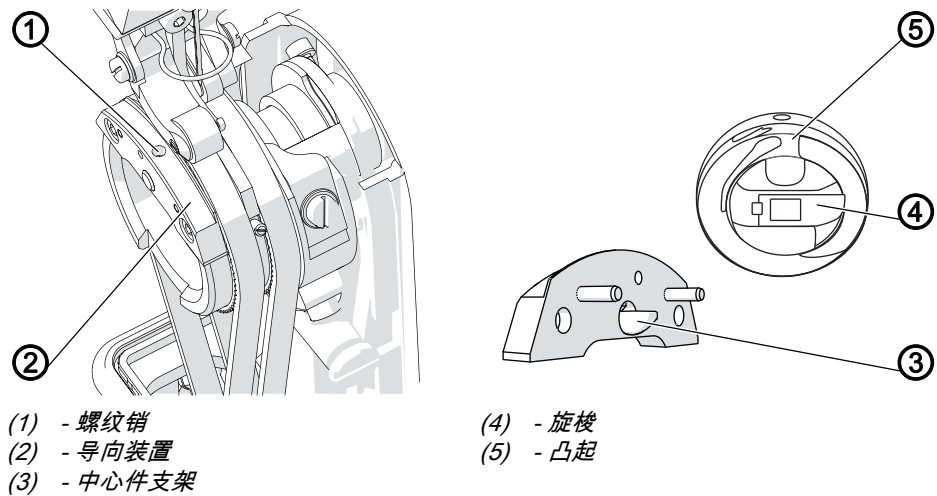
图 12: 设置中心件支架上的缝线通道
