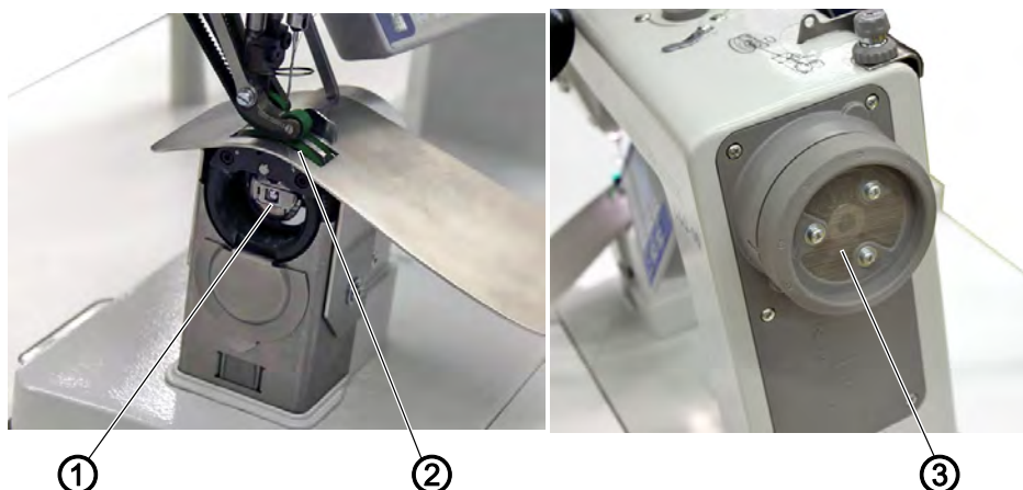
图 87: 清洁
