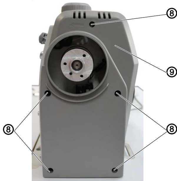
Abb. 7: Bedienfeld OP3000 demontieren (6)
