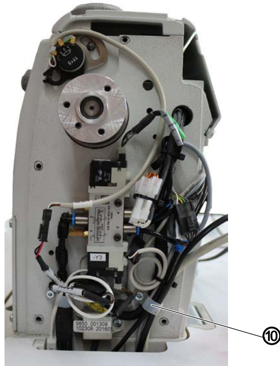
Abb. 8: Bedienfeld OP3000 demontieren (7)
