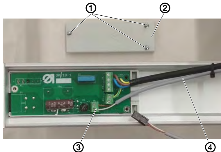
Obr. 1: Montáž osvětlení 1
