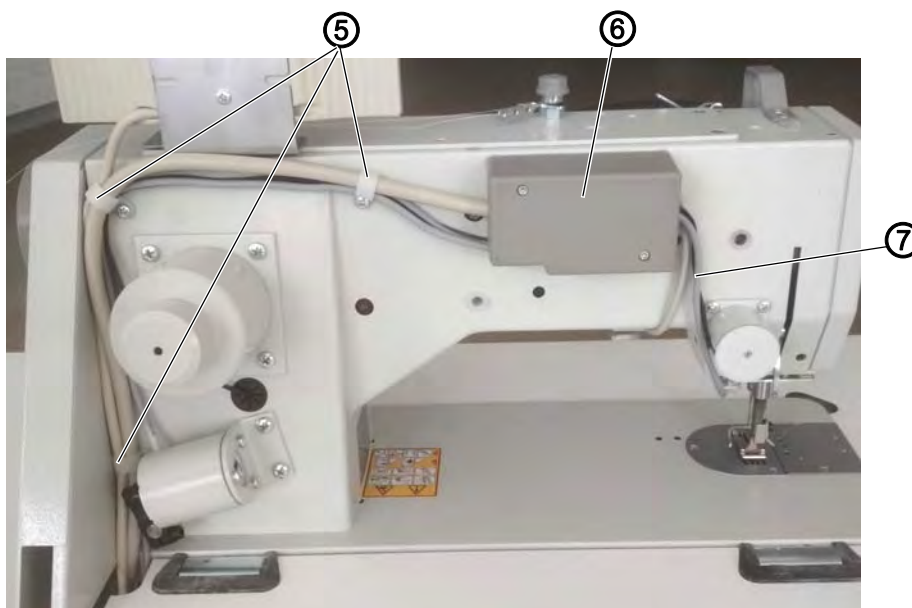
Obr. 2: Montáž osvětlení 2
