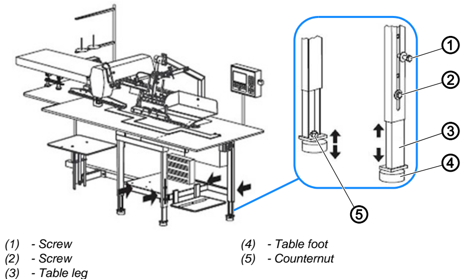
Fig. 26: Aligning the stand
