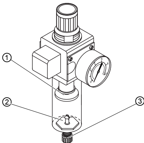
图 32: 排出冷凝水
