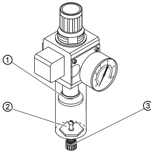
图 33: 清洁滤芯
