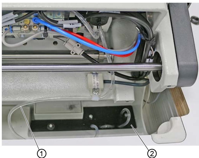
图 45: 安装吸油管路
