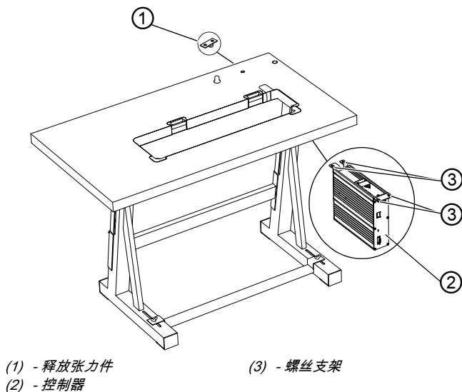
图 46: 安装控制器
