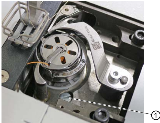
图 30: 检查旋梭润滑系统
