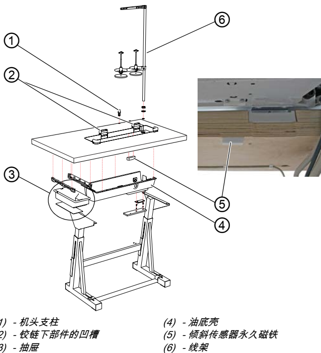
图 35: 完成工作台板
