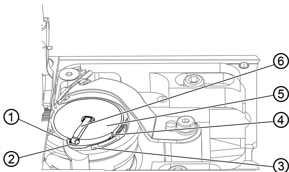
图 13: 更换梭芯线梭芯 (1)
