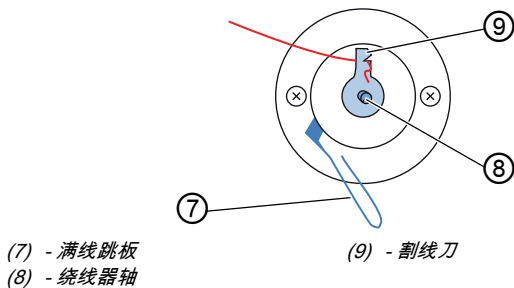
图 12: 穿入梭芯线 (3)
