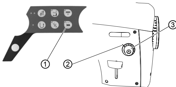
图 21: 设定线迹长度
