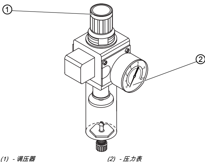
图 53: 设置工作压力
