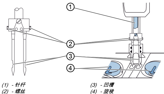
图 4: 在双针机型装入或更换机针
