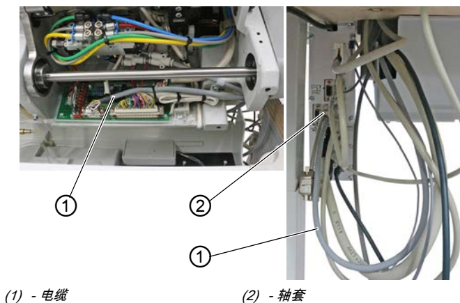
图 47: 连接控制器
