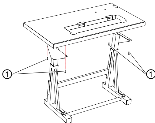
图 36: 工作台板固定至机架
