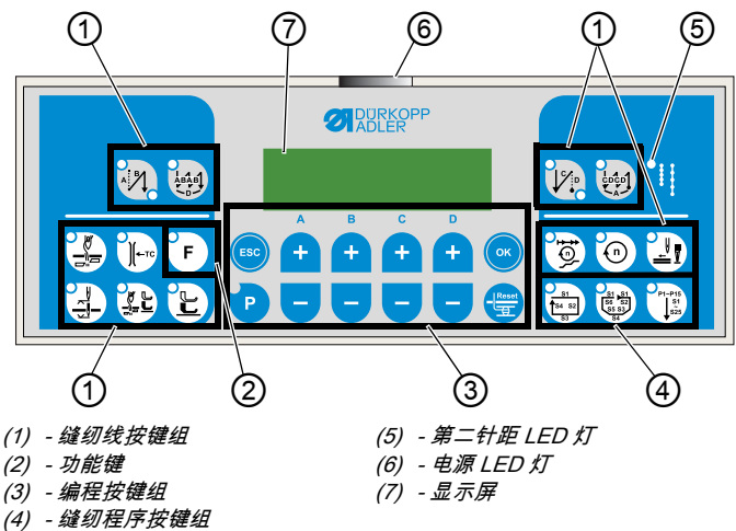
图 25: 操作面板 OP1000 (1)
