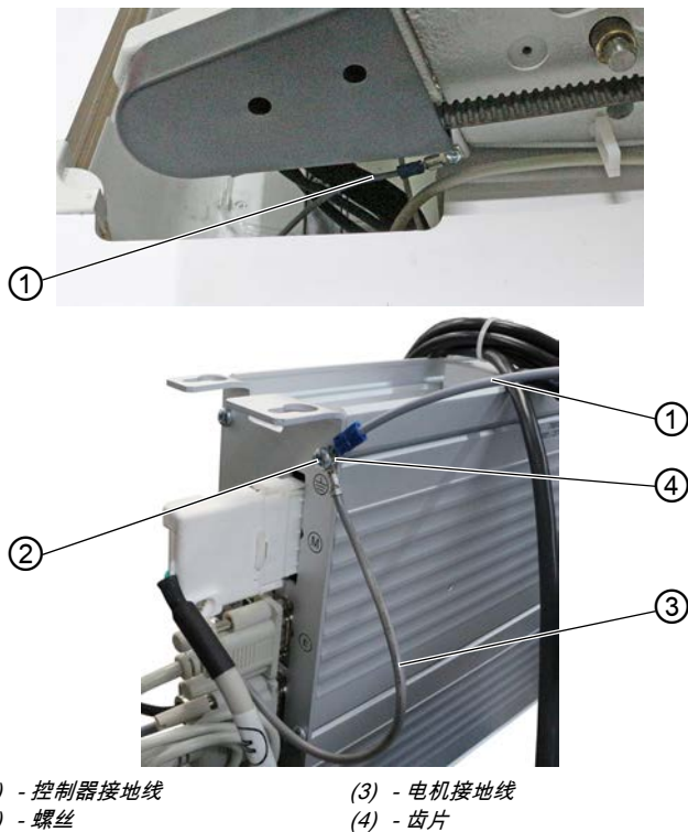
图 48: 建立电位补偿
