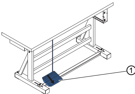
图 18: 抬起缝纫压脚
