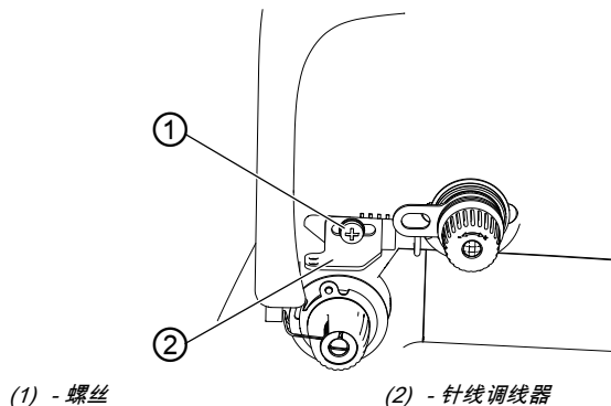
图 17: 设置针线调线器
