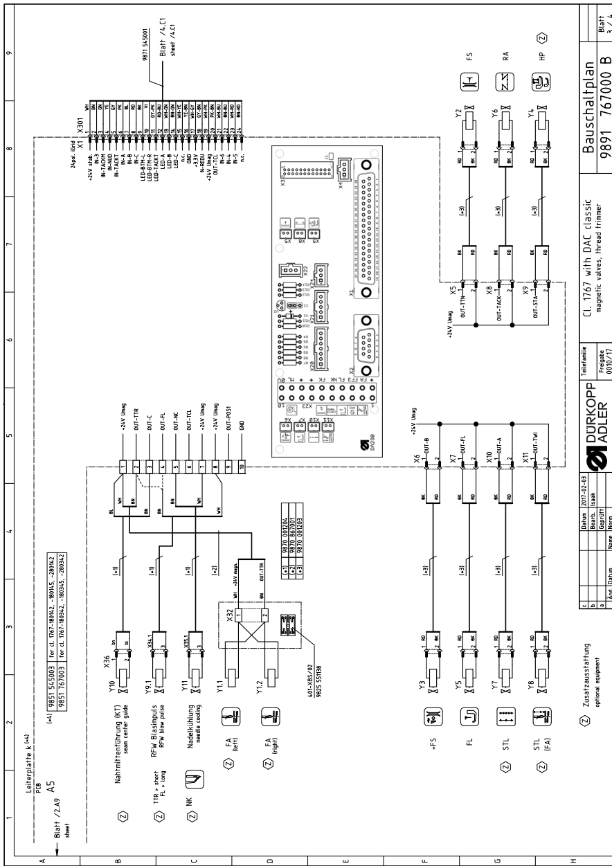
图 57: 接线图 (3)
