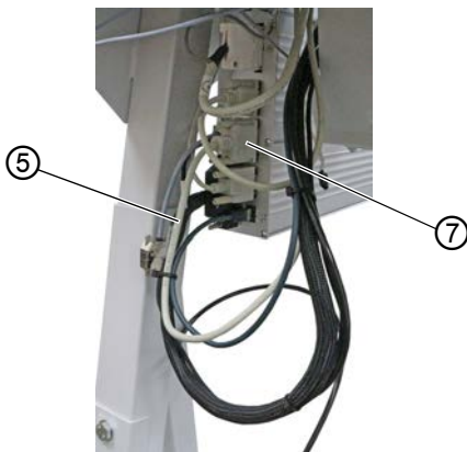
图 44: 安装操作面板 (2)
