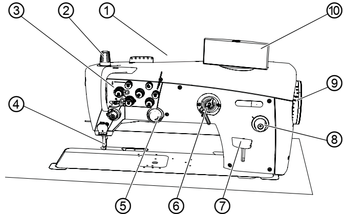
图 1: 机器组件
