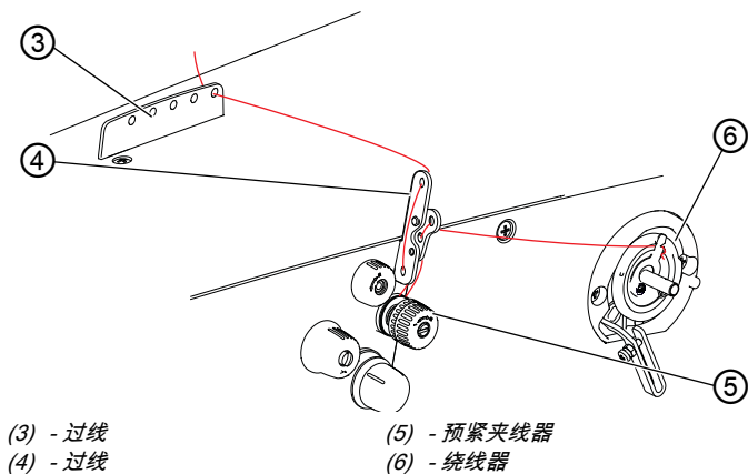
图 11: 穿入梭芯线 (2)
