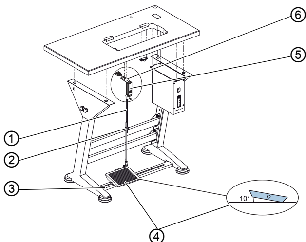
图 38: 安装踏板和额定值编码器
