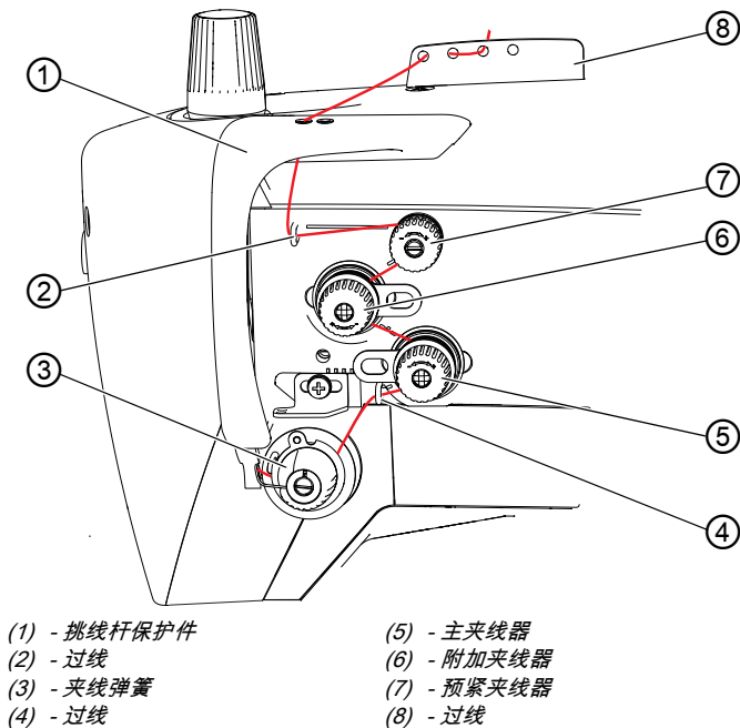
图 6: 在单针机型 (1) 穿针线
