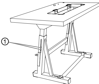
图 37: 调整工作高度
