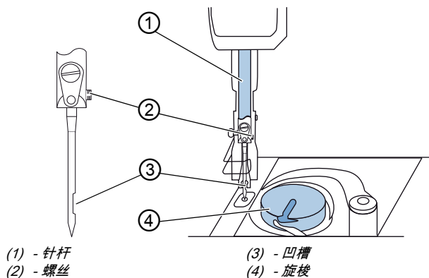
图 3: 在单针机型装入或更换机针
