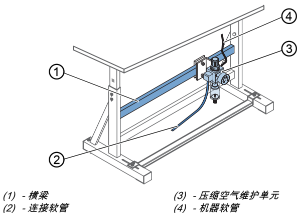
图 52: 安装压缩空气维护单元
