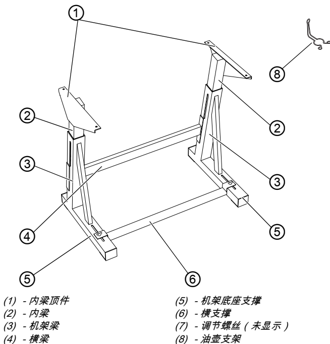
图 34: 安装机架
