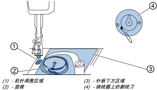
图 27: 特别需要清洁的位置
