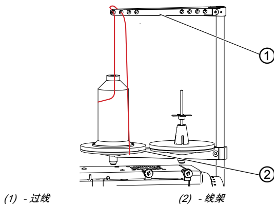
图 5: 穿针线
