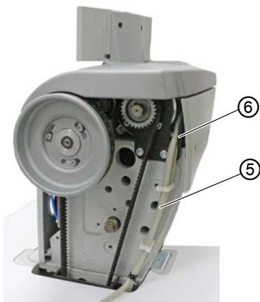
图 43: 安装操作面板 (3)
