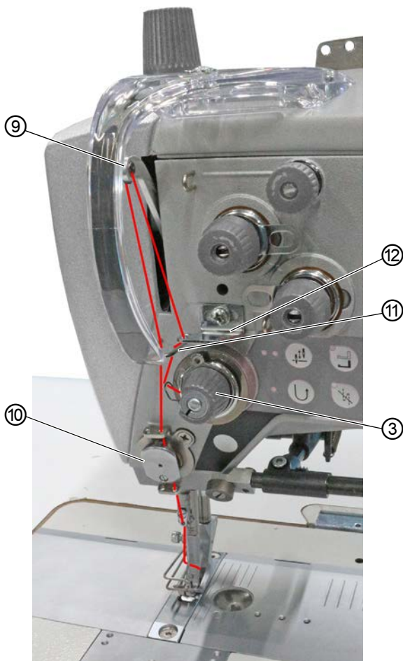
图 7: 在单针机型 (2) 穿针线
